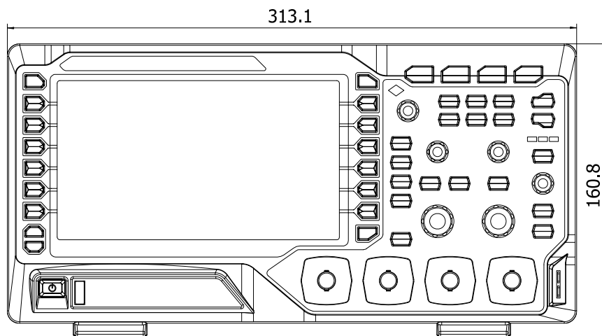
Рис. 0-1 Вид спереди
