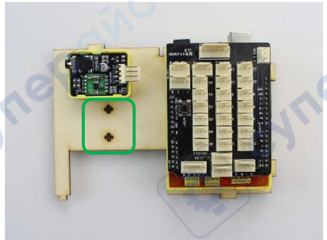
Установите модуль FM-радио на панель ①.
