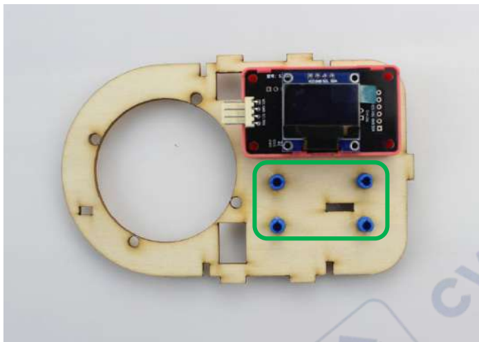
Установка клавиатуры AD на панели ②
