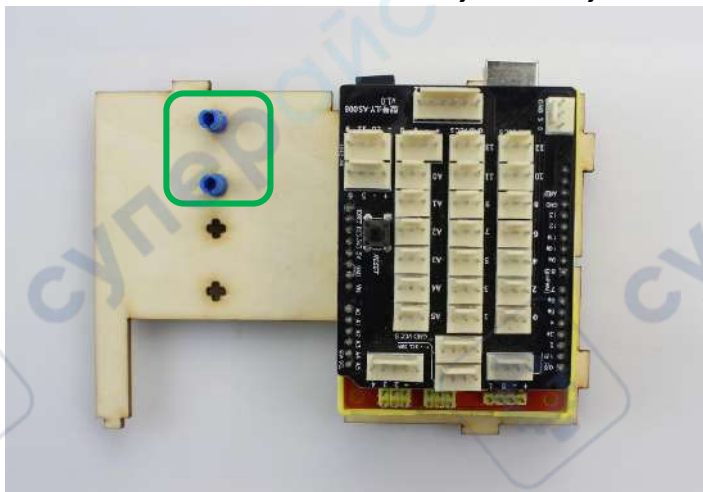
Установите модуль FM-радио на панель ①.
