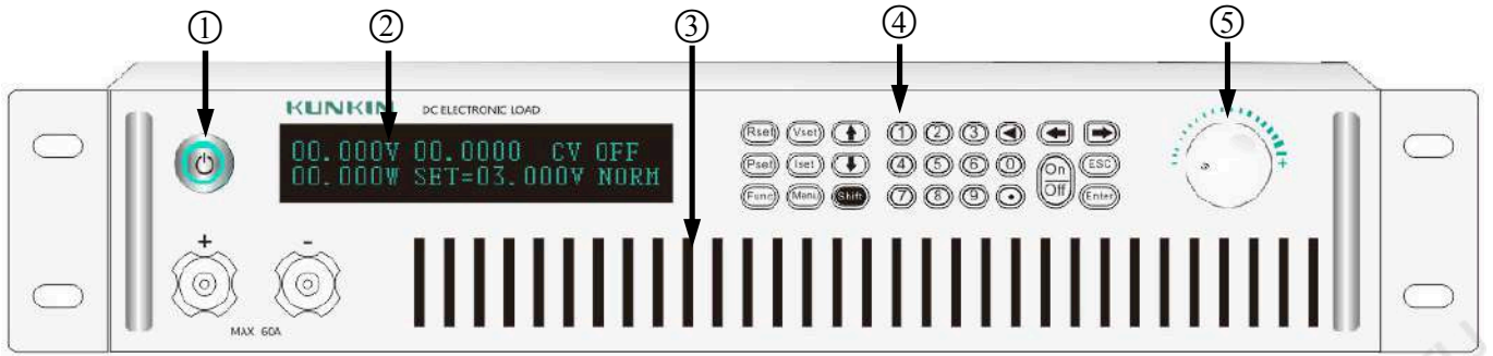
① 电源开关 ② 显示屏 ③ 散热窗口 ④ 键盘 ⑤ 编码旋钮
