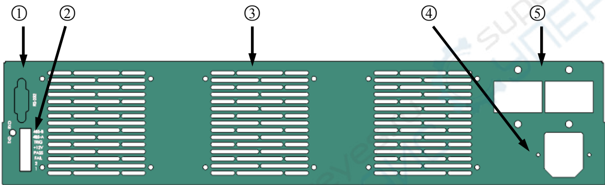
① RS232通讯接口 ② 功能接口 ③ 散热窗口 ④ 交流供电插座 ⑤ 输入接线端子
