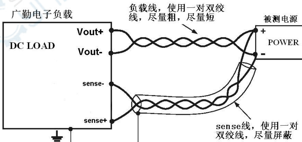
电子负载电压远端测量接线示意图
