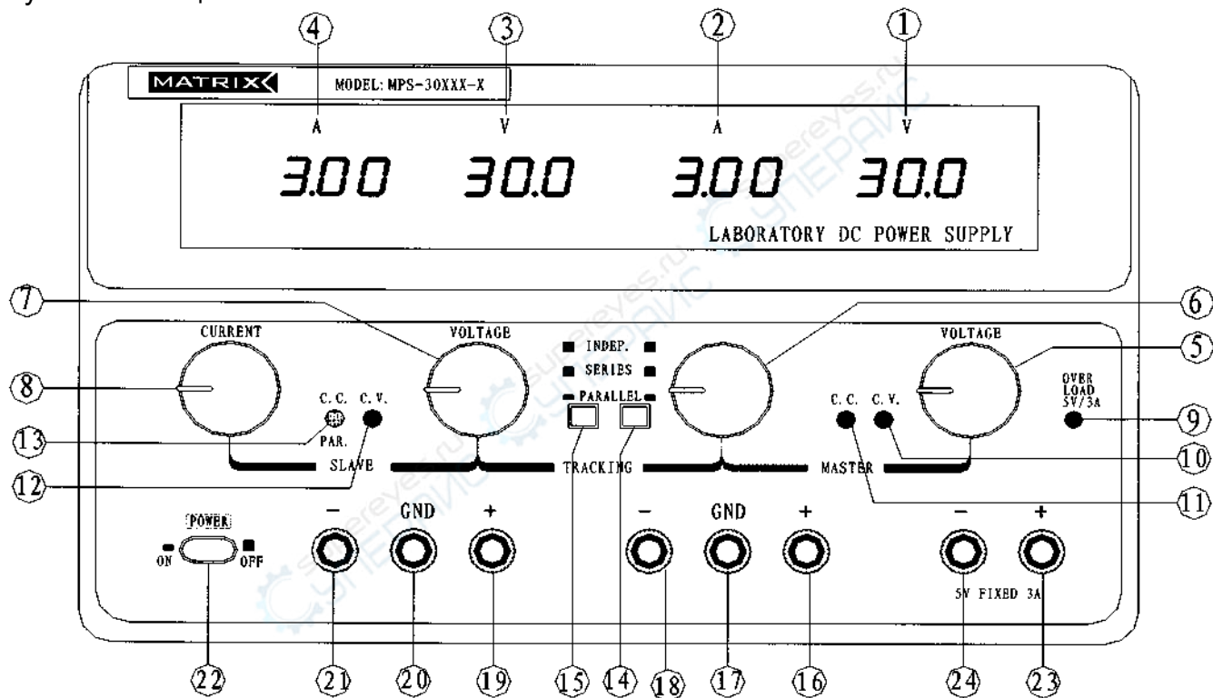
Рисунок 3-1. Лицевая панель
