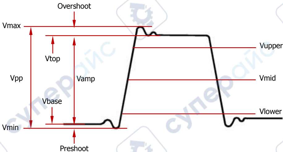
Figure 6-2 Voltage Parameters
