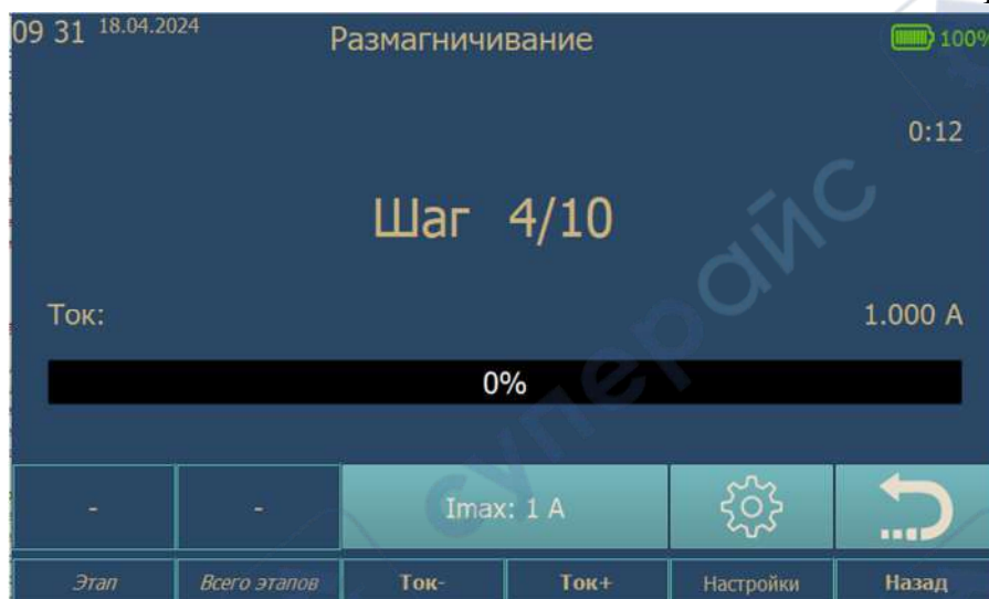
Рис. 5. Режим размагничивания
