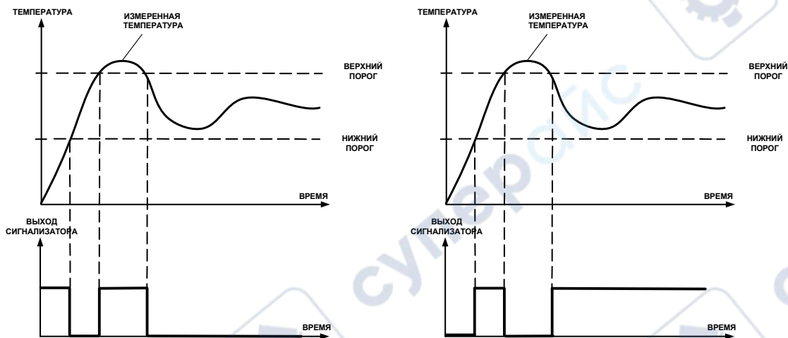
Рисунок 3.9 Функция вида f = НП+ВП , слева – сигнализация выхода измеряемого параметра за диапазон, справа – тоже с инверсией, сигнализация, что измеряемый параметр находится в диапазоне
