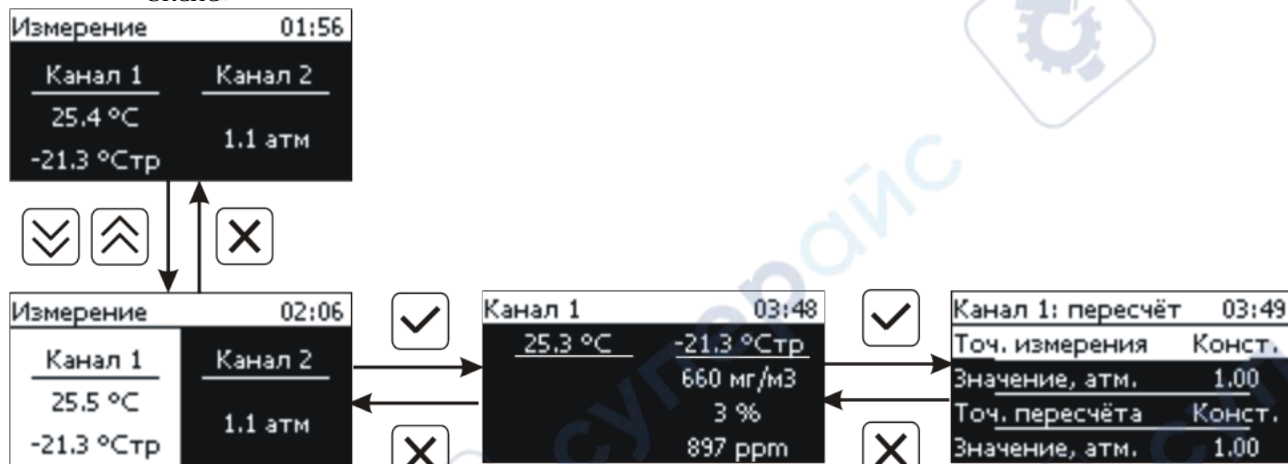
Рисунок 6.24 переход к экрану настроек пересчета влажности.
