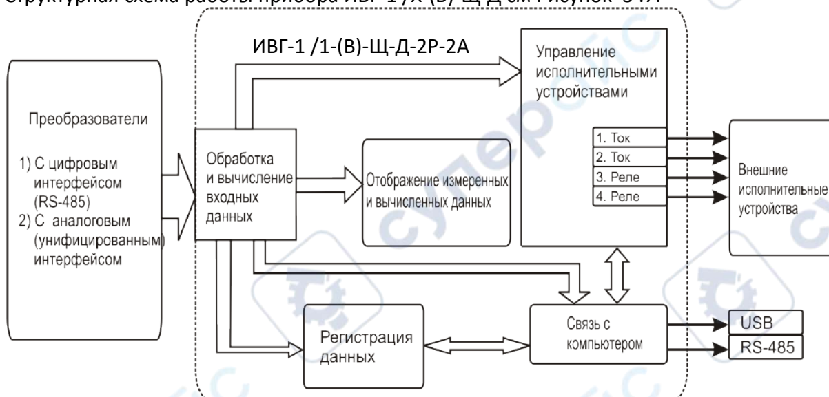
Рисунок 3.7 Структурная схема работы прибора
