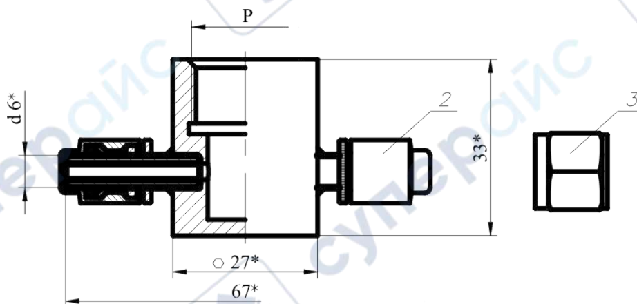
Рисунок В2 Проточная камера со штуцерами d=6
