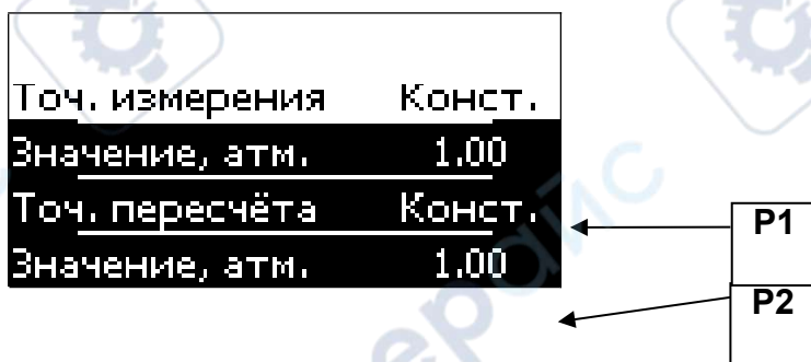
Рисунок 6.25 Вид экрана настройки пересчета влажности
