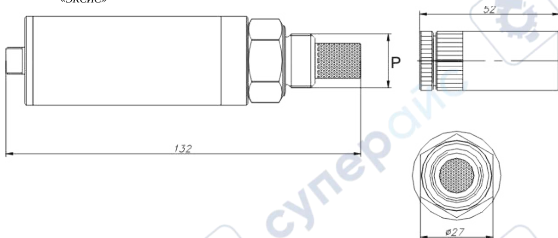
Рисунок 3.12 Внешний вид измерительного преобразователя ИПВТ-08
