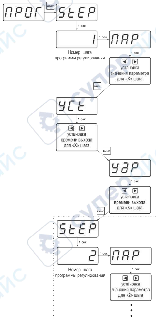
Рисунок 6.34 Программа регулирования
