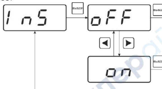
Рисунок 6.35 Схема меню инверсии логики работы канала управления OFF - прямое управление; On - инверсное управление.
