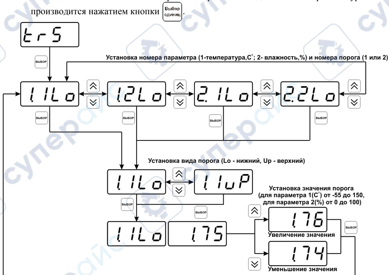
Рисунок 6.11 Задание порогов по влажности и температуре
