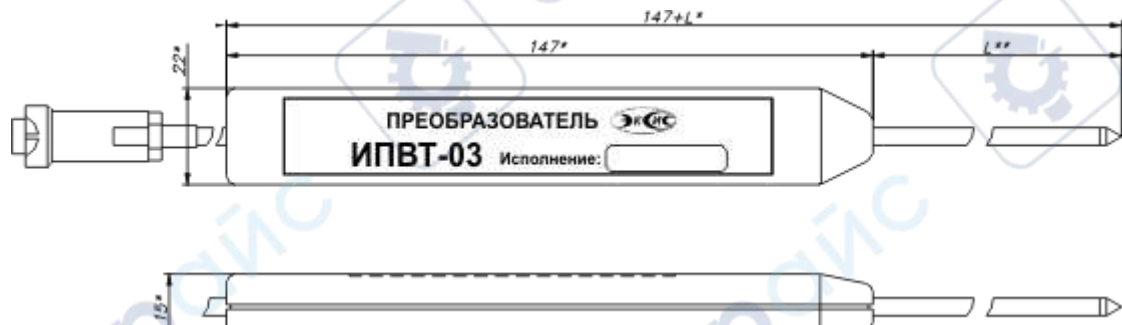
Рисунок В4 Измерительный преобразователь ИПВТ-03-05
