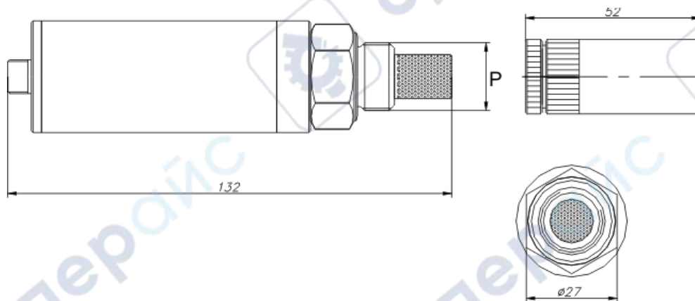
Рисунок 3.18 Внешний вид измерительного преобразователя ИПБТ-08
