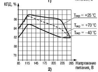
Рисунок 7 - График зависимости КПД от напряжения питания и температуры окружающей среды: (1) БП30А-12С, (2) БП30А-24С
