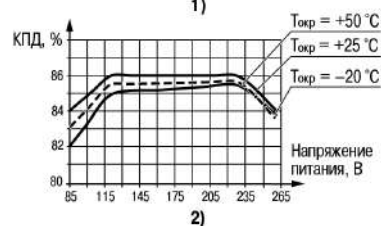
Рисунок 7 - График зависимости КПД от напряжения питания и температуры окружающей среды: (1) БП60А-12, (2) БП60А-24
