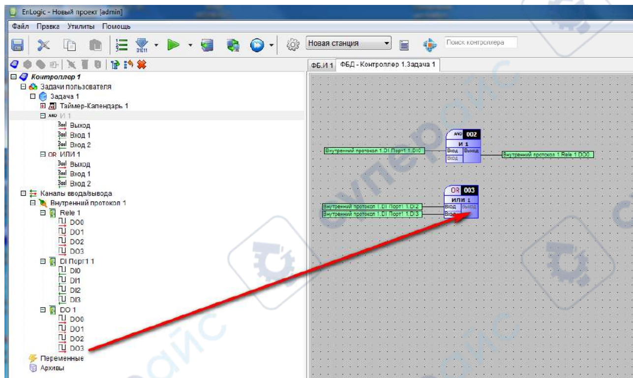
Рисунок 4.9 – Привязка сигнала к функциональному блоку
