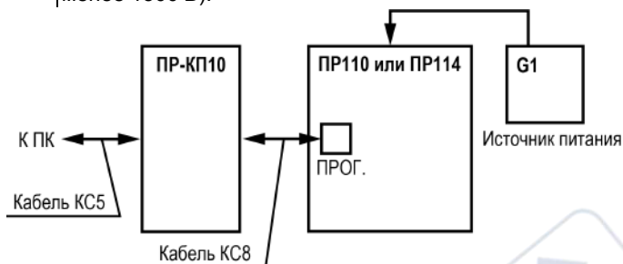
Рисунок 4 – Схема подключения ПР110/ПР114 к ПК
