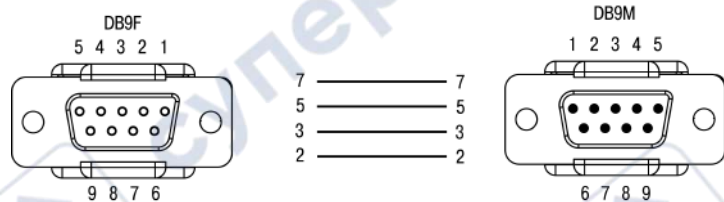
Рисунок 6 – Кабель КС5
