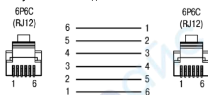
Рисунок 5 – Кабель КС8
