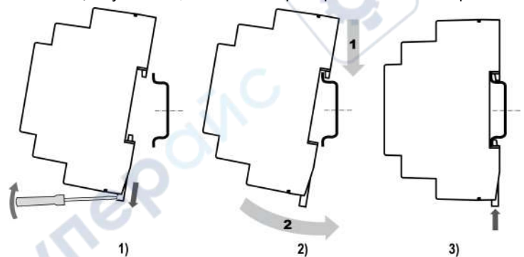
Рисунок 3 – Монтаж прибора
