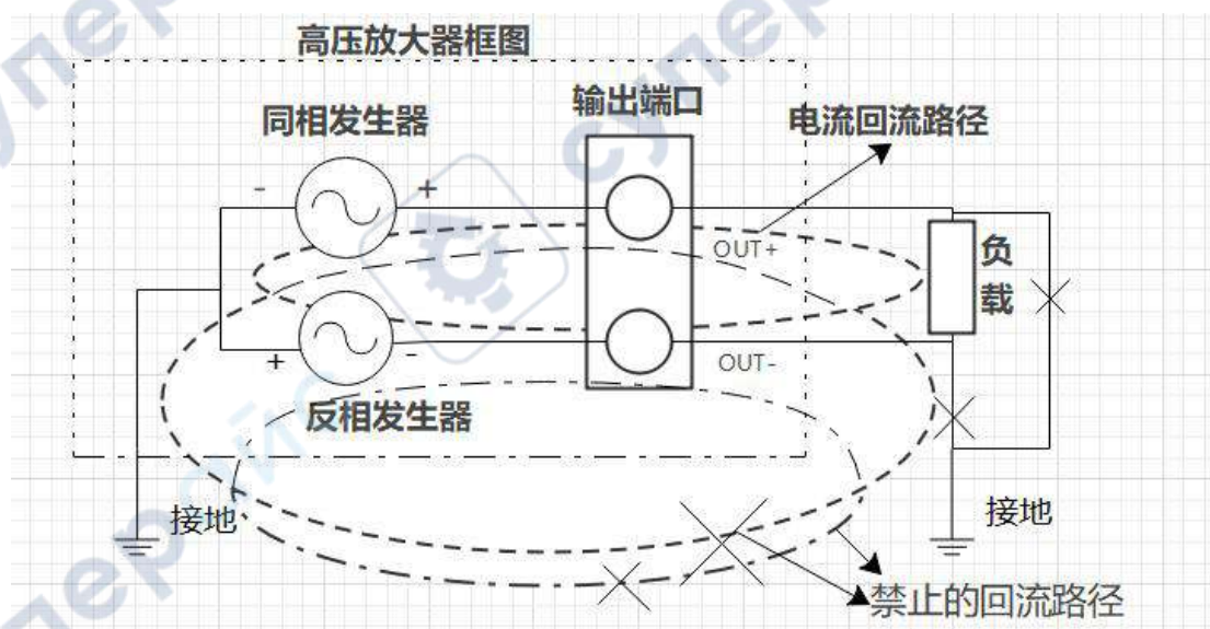
图 1 差分输出
