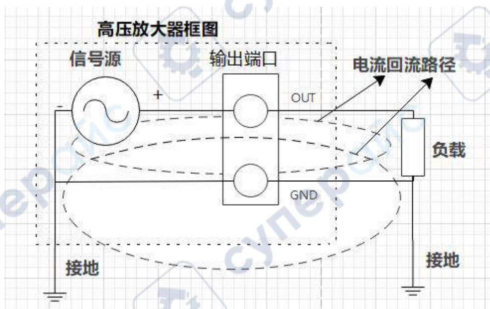
图 2 单端输出（可接地）：HA-205/HA-400/HA-405/HA-800/HA-805
