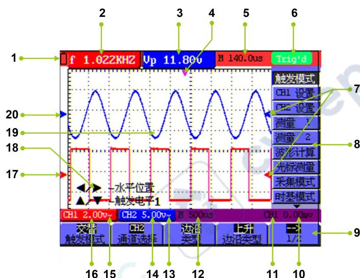
图 4：示波器界面
