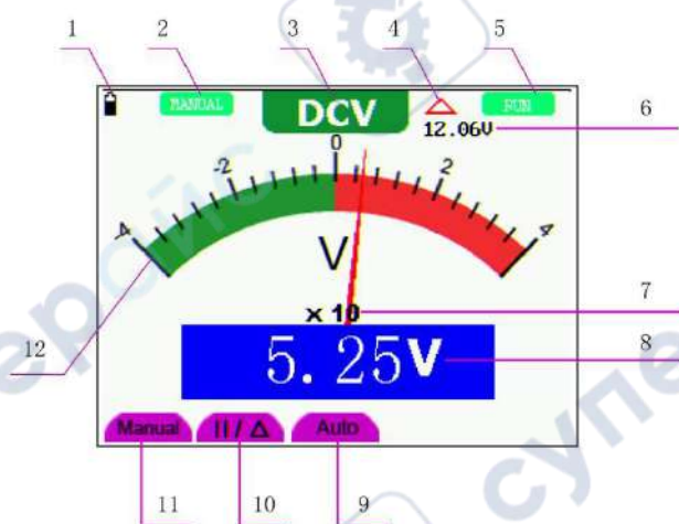
图 5：万用表界面
