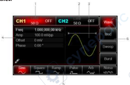
Рис. 6 Описание дисплея
