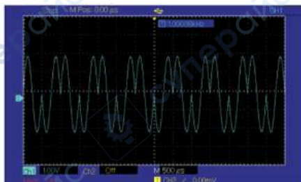
Рис. 81 Осциллограмма сформированного сигнала с балансной амплитудной модуляцией
