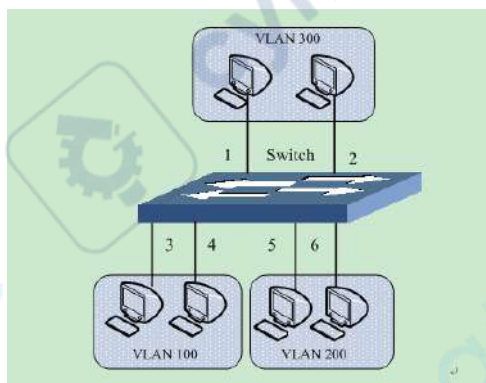
Рис. 51. Типовая конфигурация PVLAN
