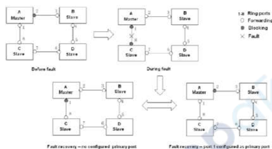
Рис. 123. Пример работы ST-Ring
