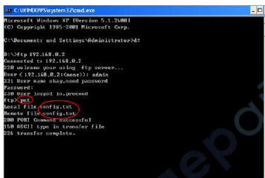
Рис. 82. Выгрузка файла из ПК по FTP
