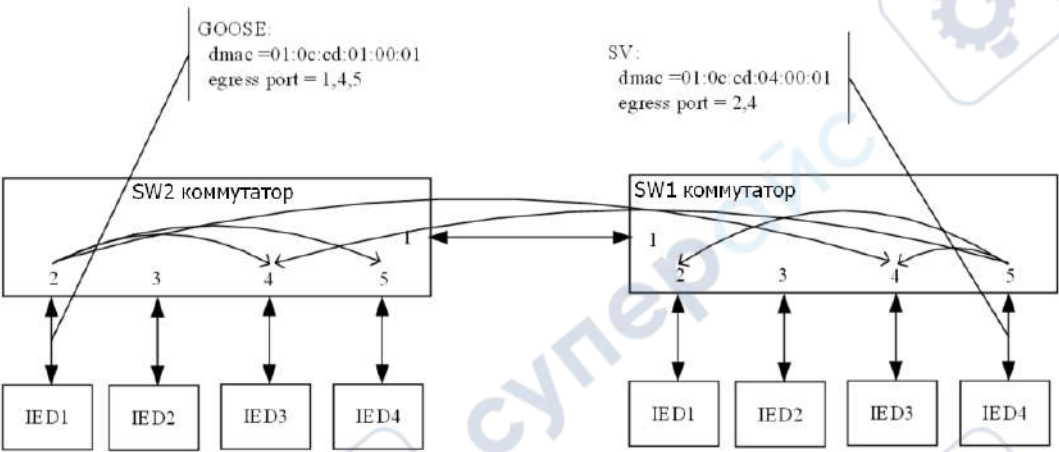
Рис. 244. Пример топологии
