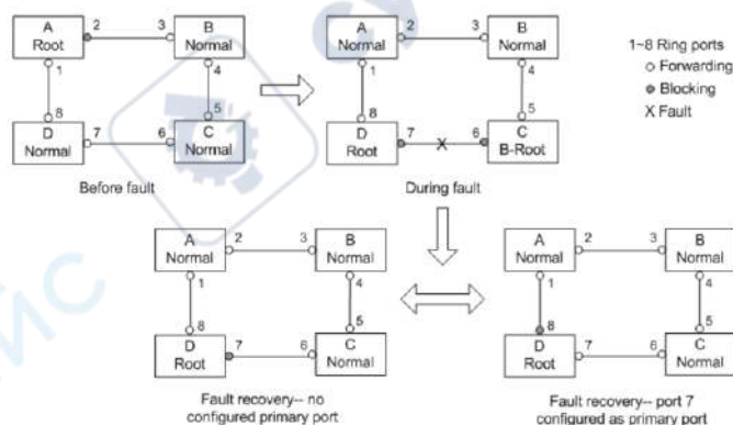
Рис. 136. Процесс восстановления после сбоя
