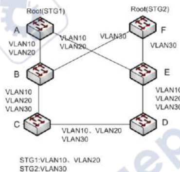
Рис. 137. Пересылка пакетов по разным VLAN
