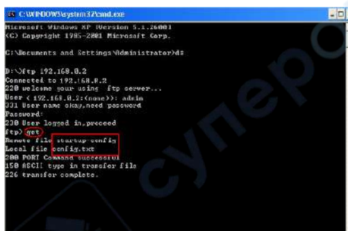
Рис. 81. Загрузка файла в ПК по FTP
