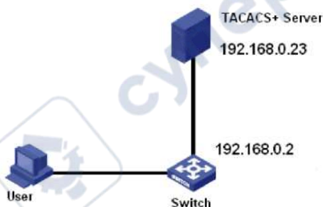
Рис. 275. Пример конфигурации
