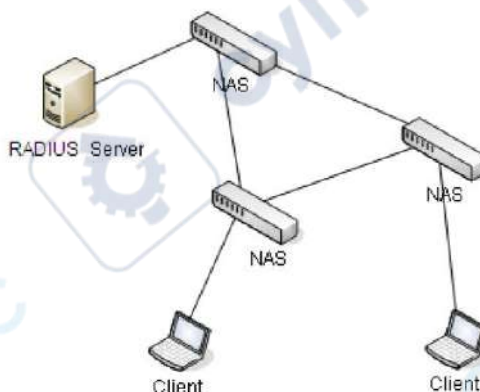
Рис. 277. Структура RADIUS
