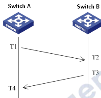
Рис. 261. Пример работы NTP
