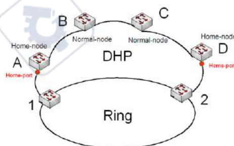
Рис. 139. Пример применения DHP
