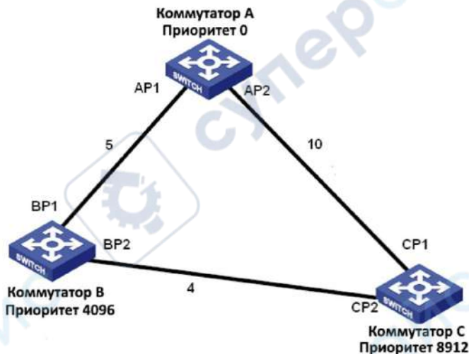
Рис. 135. Пример конфигурации
