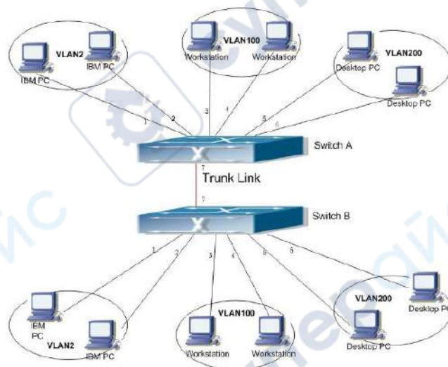
Рис. 45. Типовая конфигурация
