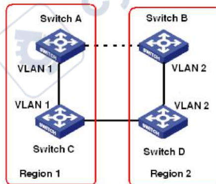
Рис. 157. Пример подключения
