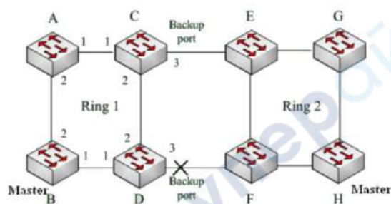
Рис. 125. Пример реализации ST-Ring VLAN
