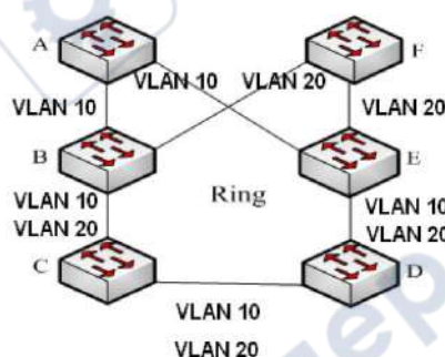
Рис. 124. Пример ST-Ring VLAN
