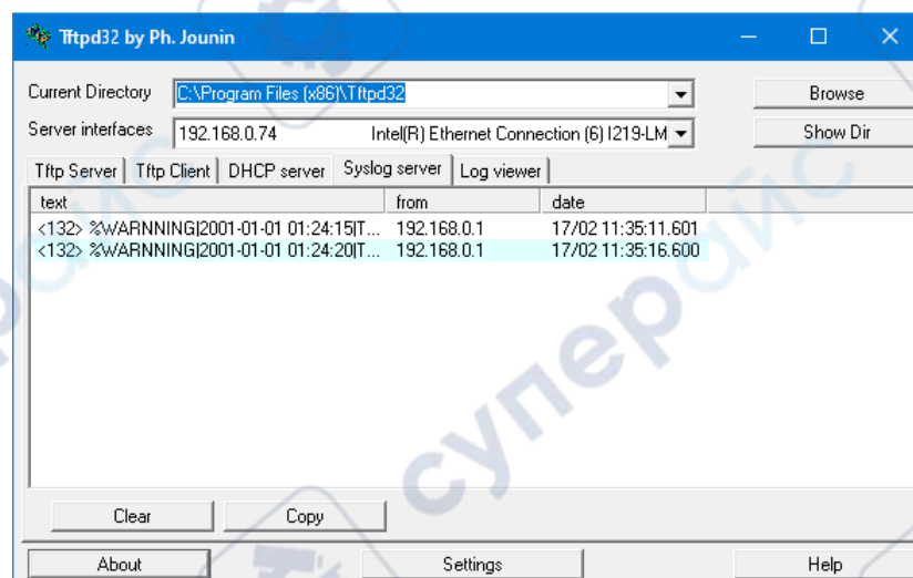
Рис. 185. Отображение информации в Syslog Server
