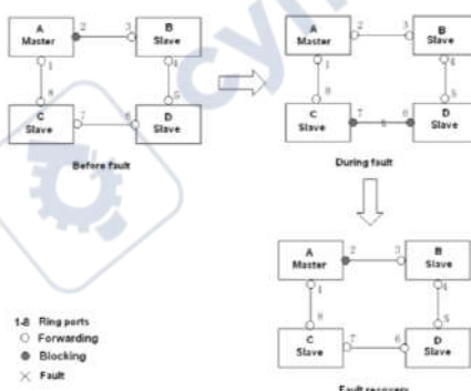
Рис. 122. Пример работы ST-Ring
