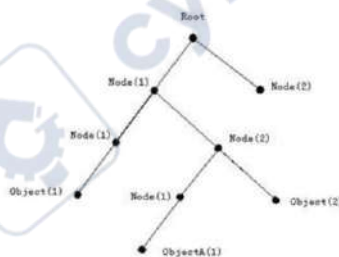
Рис. 107. Структура MIB
