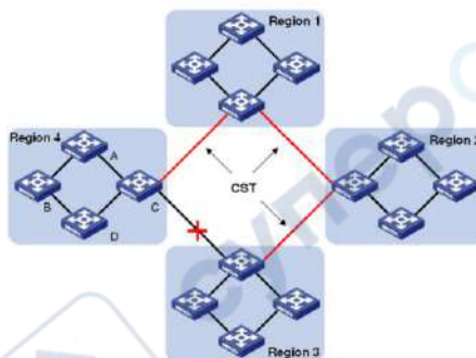
Рис. 158. MSTP концепция
