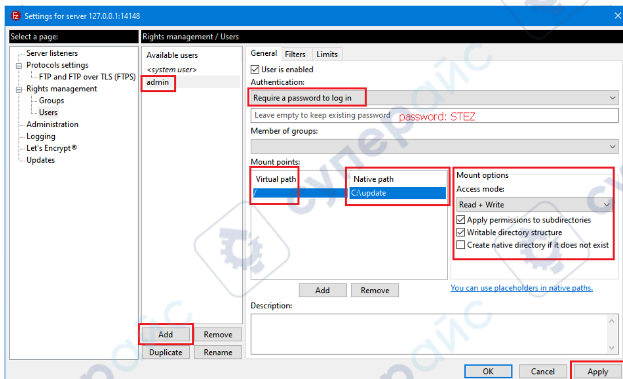
Рис. 12. Создание нового FTP пользователя
