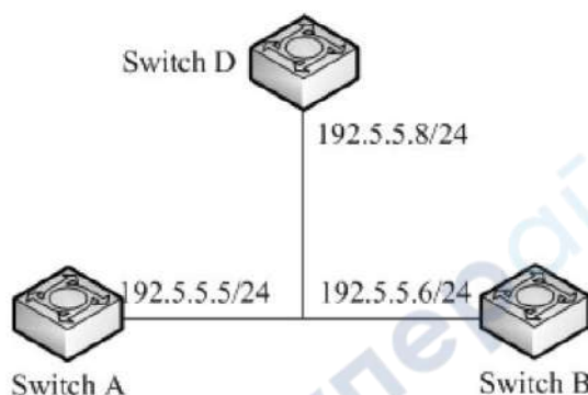
Рис. 269. Настройка многоадресного режима
