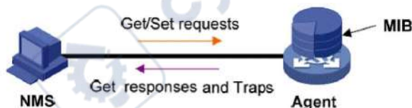
Рис. 106. Взаимосвязи между NMS, агентом и MIB
