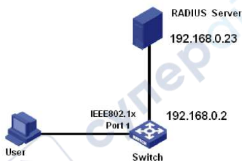
Рис. 280. Типовая конфигурация
