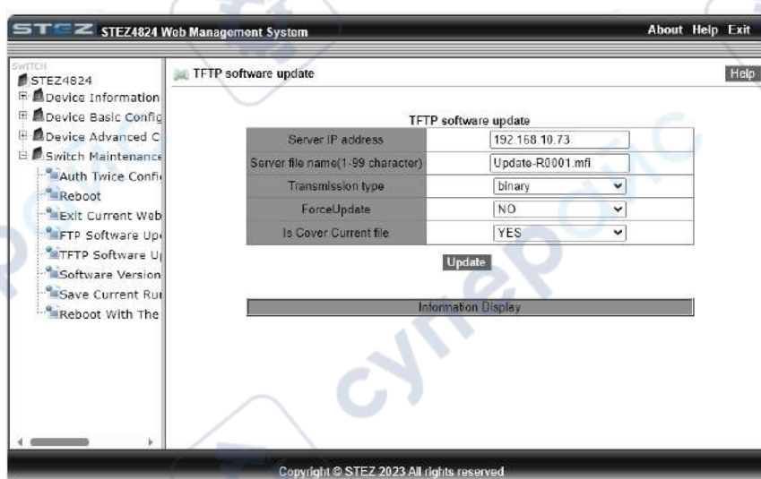
Рис. 18. Обновление ПО через TFTP
