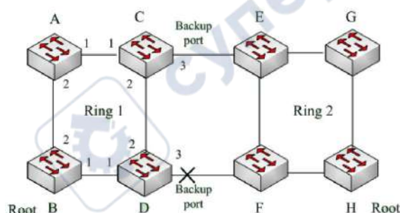
Рис. 138. Резервирование двух колец
