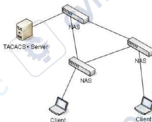
Рис. 271. Структура TACACS+
