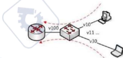
Рис. 50. PVLAN пример настройки
