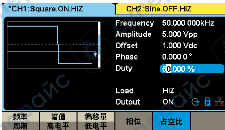
图 3-2 输出方波
