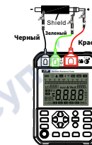
Рис. 10.1.2 Трехпроводное подключение
