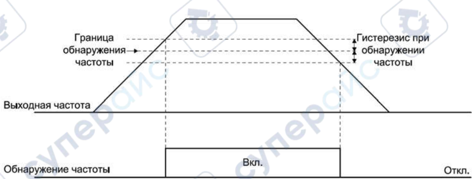
Рисунок 10.10-3 – Граница и гистерезис обнаружения выходной частоты (функций 9 и 10 параметров F06.21-F06.24)
