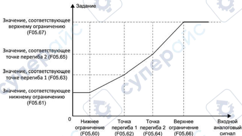
Рисунок 10.9-11. – Кривая 1 аналогового входа (аналогично для кривой 2)
