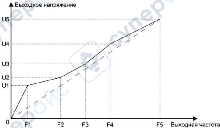
Рисунок 10.8-3. – Пользовательская характеристика U/f
