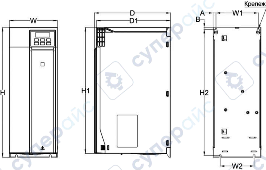
Рисунок 3.6-4 – Чертеж преобразователя частоты типоразмера В4
