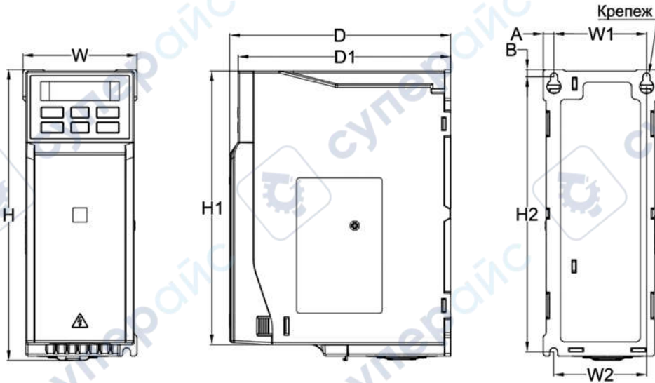
Рисунок 3.6-1 – Чертеж преобразователя частоты типоразмера В1
