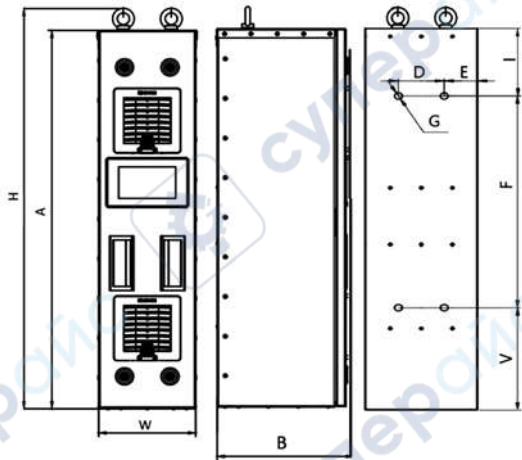
Рисунок 3.9-1. – Чертеж преобразователя частоты VF-101 HVC
