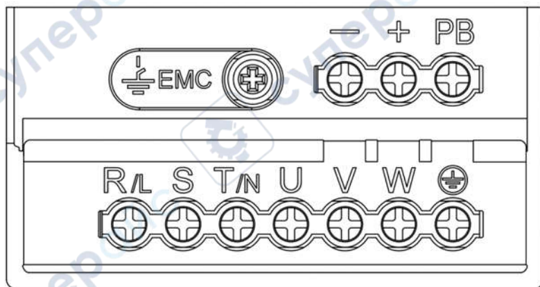
Рисунок 4.4-3. – Расположение клемм
