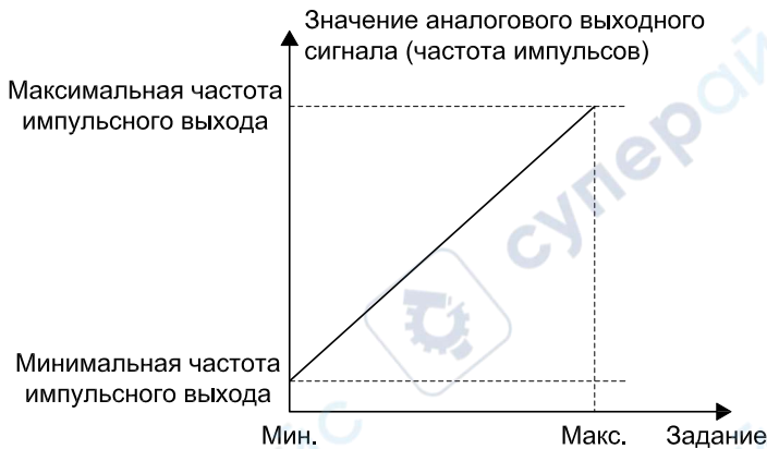
Рисунок 10.10-2 – Амплитудная характеристика импульсного выхода
