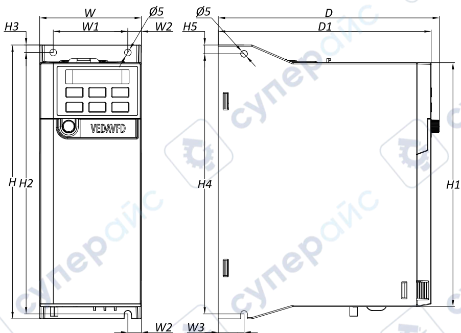
Рисунок 3.6-3 – Чертеж преобразователя частоты типоразмера А2 с защитной крышкой
