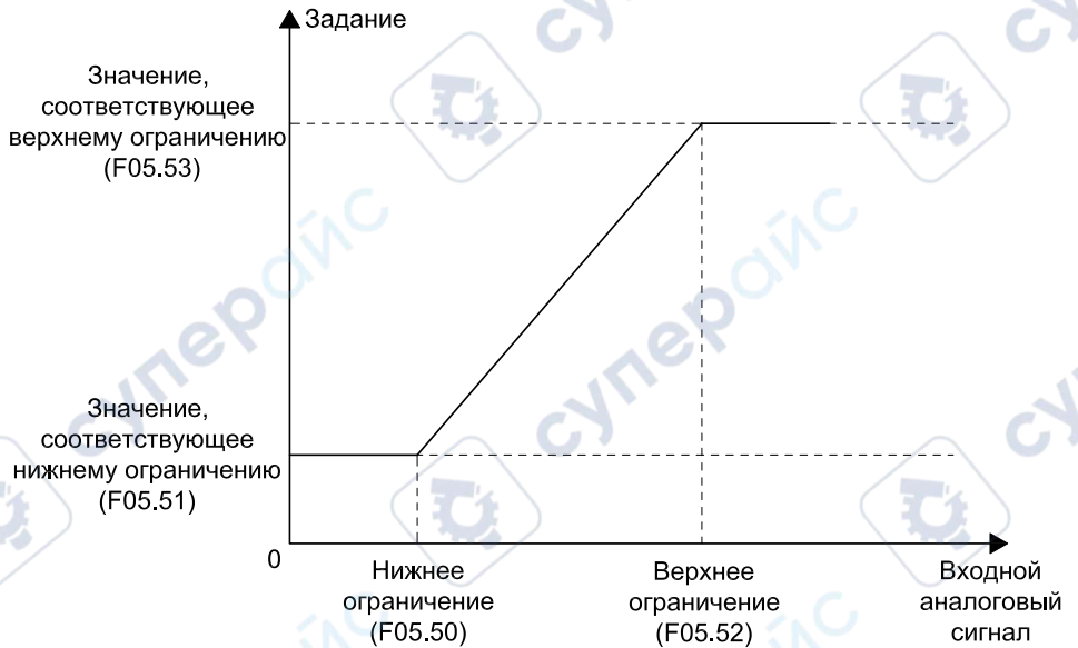
Рисунок 10.9-10 – Линейная характеристика аналогового входа (F05.43 = 1)
