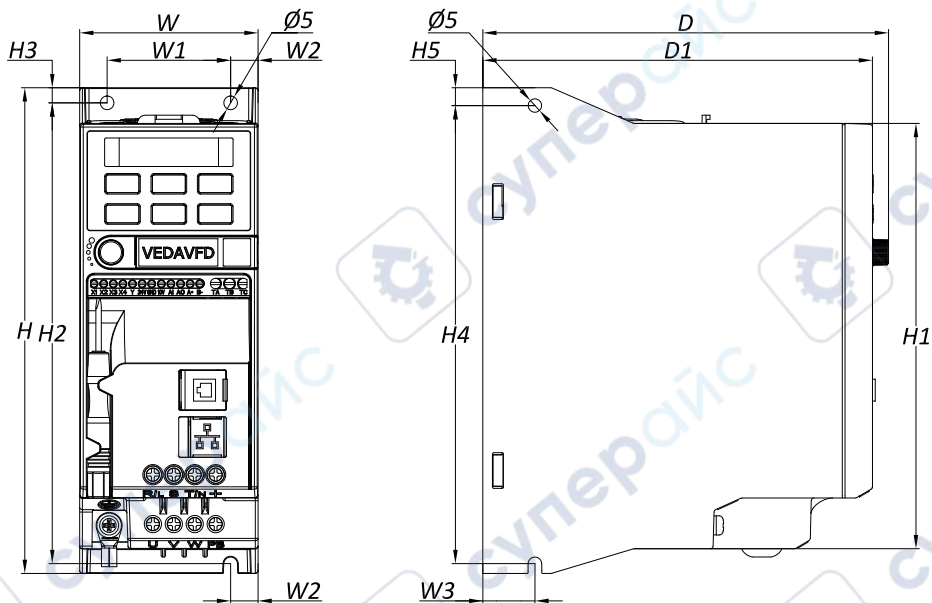
Рисунок 3.6-2 – Чертеж преобразователя частоты типоразмера A1 без защитной крышки
