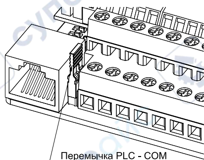
Рисунок 4.7-3. Схема подключения перемычек «+24 В», «PLC», «COM» для мощностей 7,5-22 кВт
