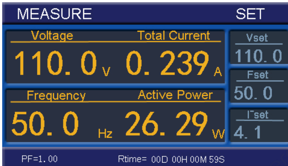
图 7 电源启动态
