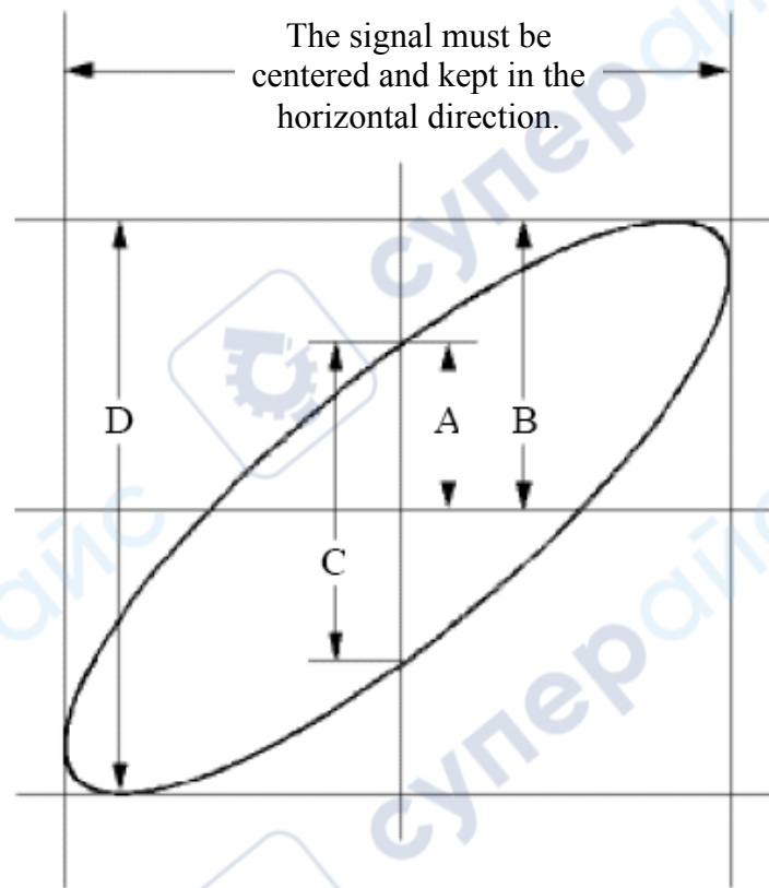
Fig.6-6 Lissajous Graph
