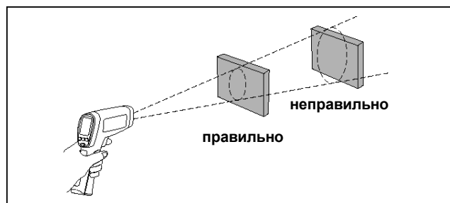
Рисунок 7. Поле обзора.
