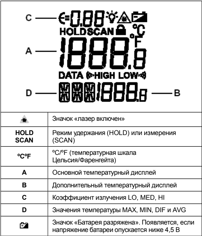
Рисунок 3. Дисплей термометра
