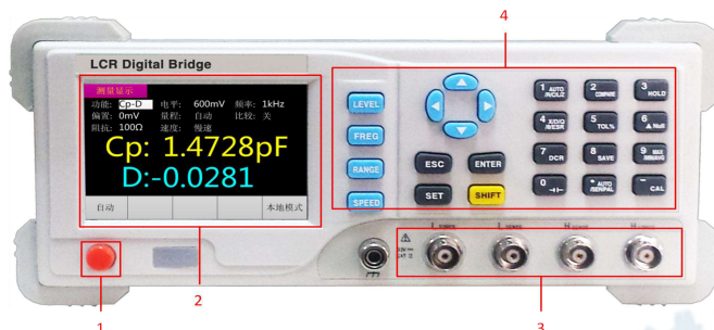
图 3-1 前面板示意图
