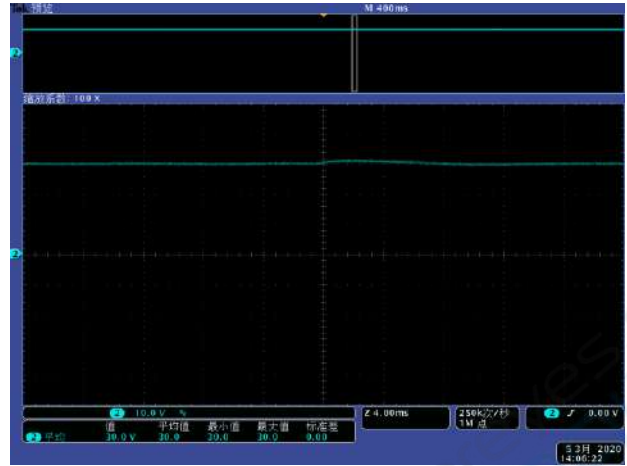
50%到 10%负载变动情况下，动态响应波形
