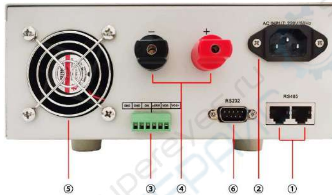
①RS-485 通信接口 ②市电输入口 ③外部采样 控制接口 ④输出接口 ⑤风机 ⑥RS-232 通信接口
