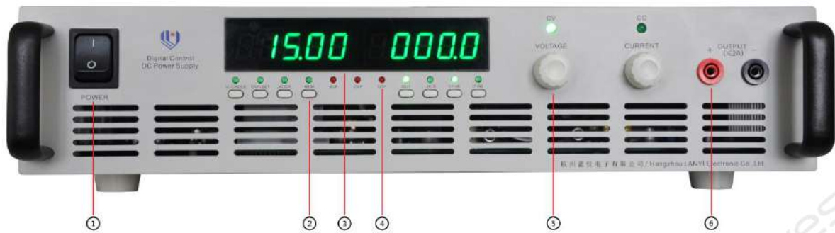
①电源开关 ②功能按键 ③数码显示区域 ④状态指示 ⑤调节区域 ⑥输出检测
