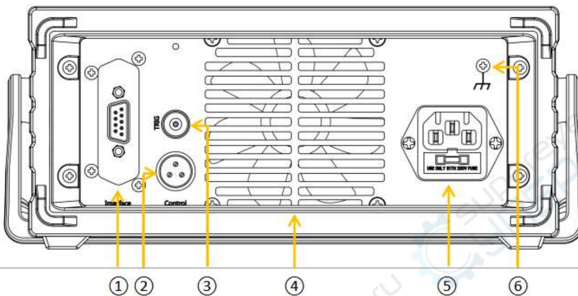
后面板图
