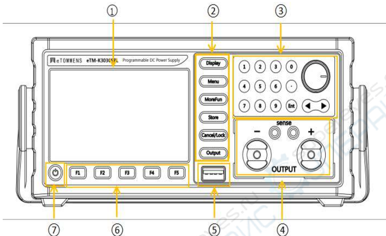
前面板图
