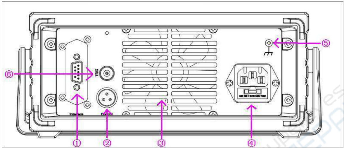
后面板图
