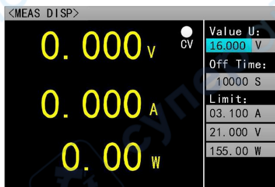
Рисунок 4.6.2. Режим стабилизации напряжения
