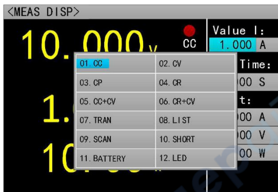
Рисунок 4.6. Активация режима стабилизации тока
