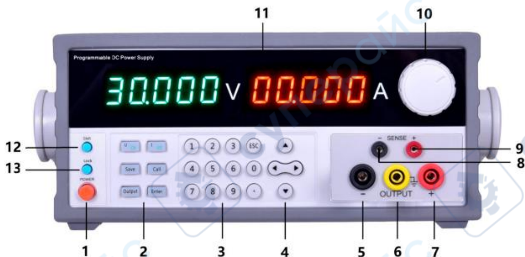
Передняя панель
