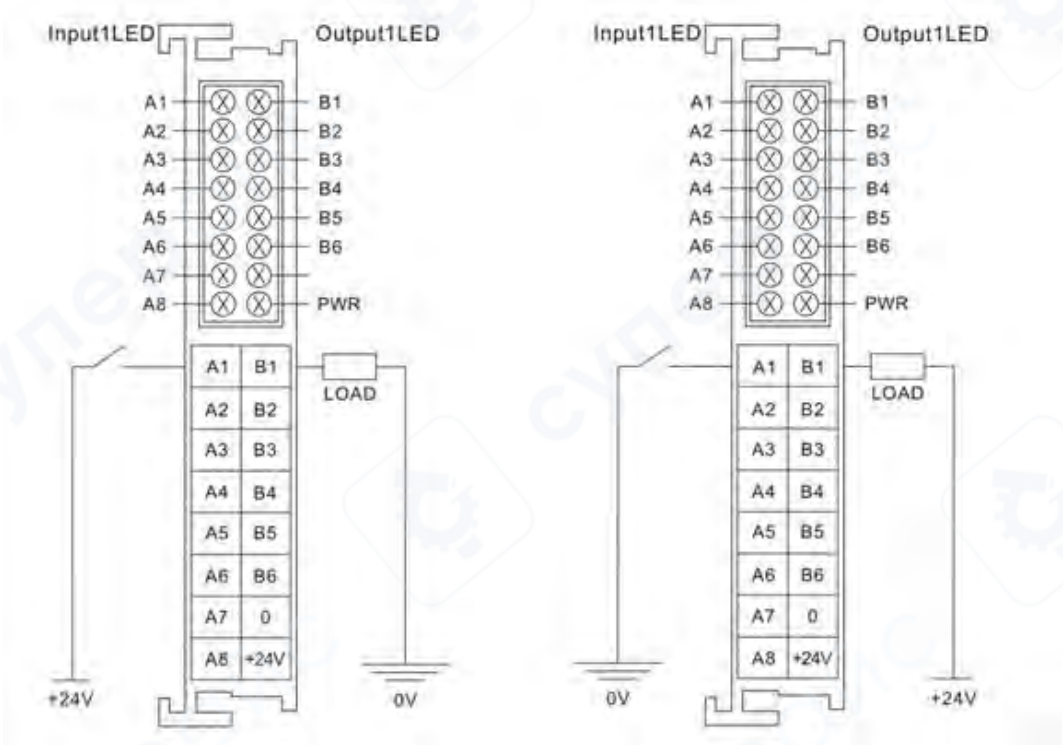
图 2.8 PNP 型接线端子排
