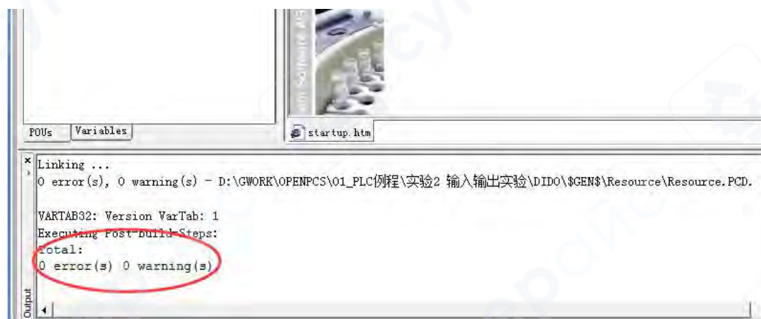
图 5.14 编译完成
