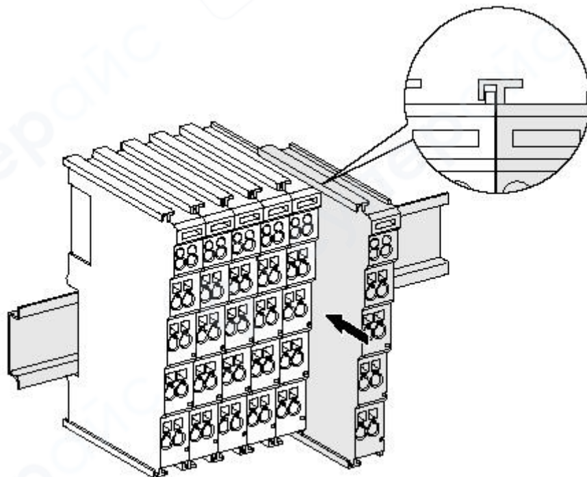
图 2.3 GCAN-PLC-IO 安装
