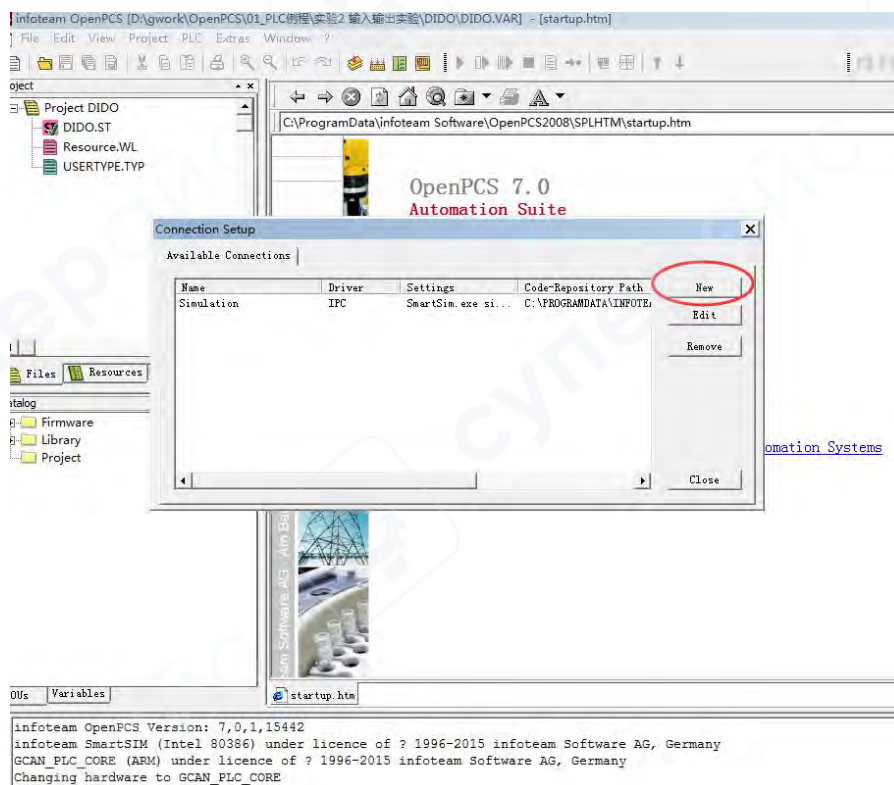
图 5.5 点击“New”
