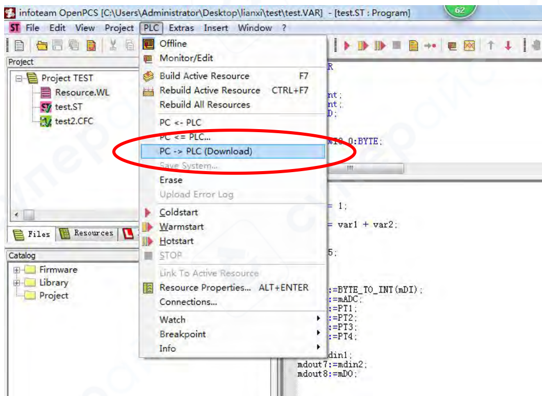
图 5.16 下载程序
