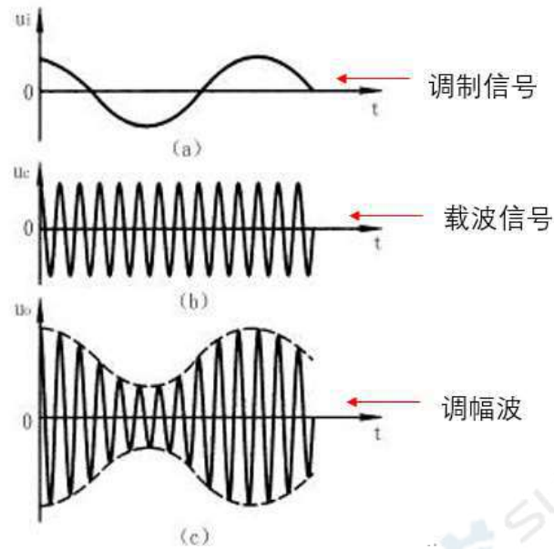
图 20.15 调幅
