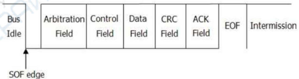
图 8.12 CAN 总线示意图
