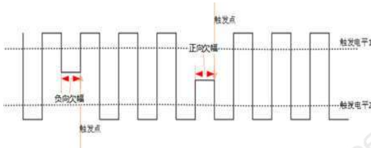
图 8.7 欠幅触发示意图
