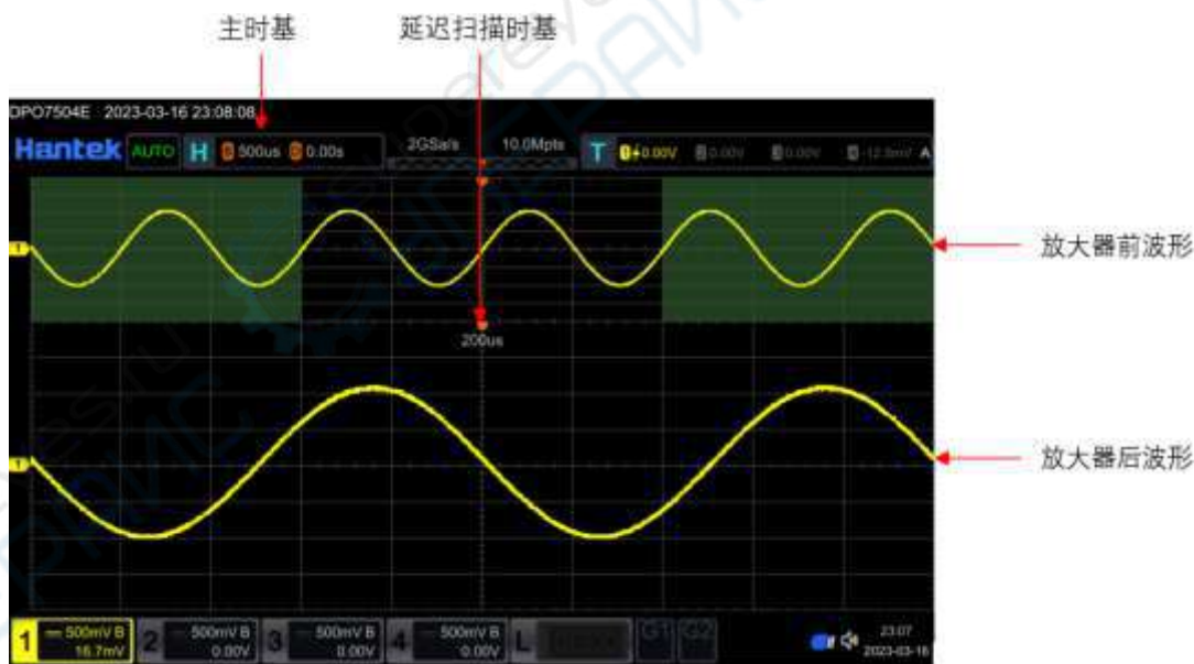
图 6.1 延迟扫描模式
