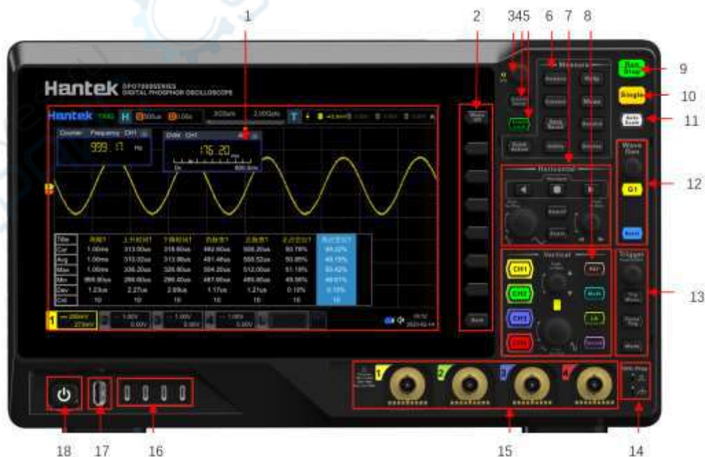
图 4.8 前面板总览
