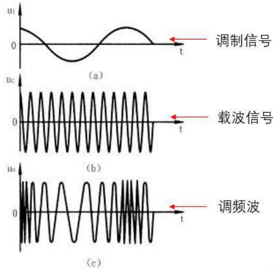
图 20.16 调频
