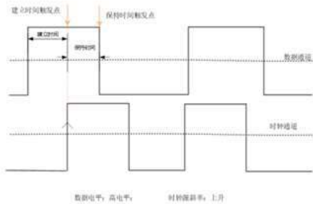
图 8.9 建立保持触发示意图
