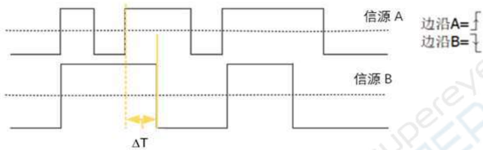
图 8.8 延迟触发示意图
