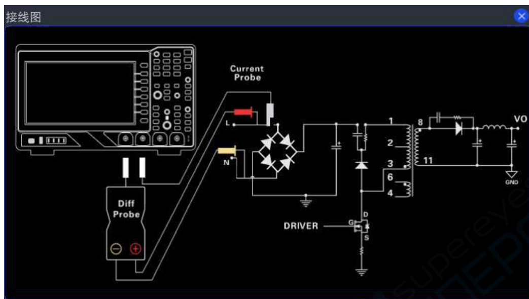
图 16.1 电源分析接线图
