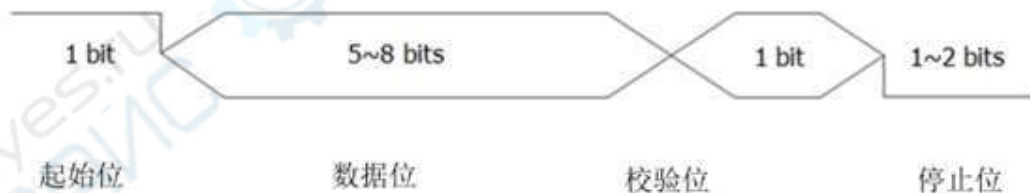
图 8.10 RS232 触发示意图
