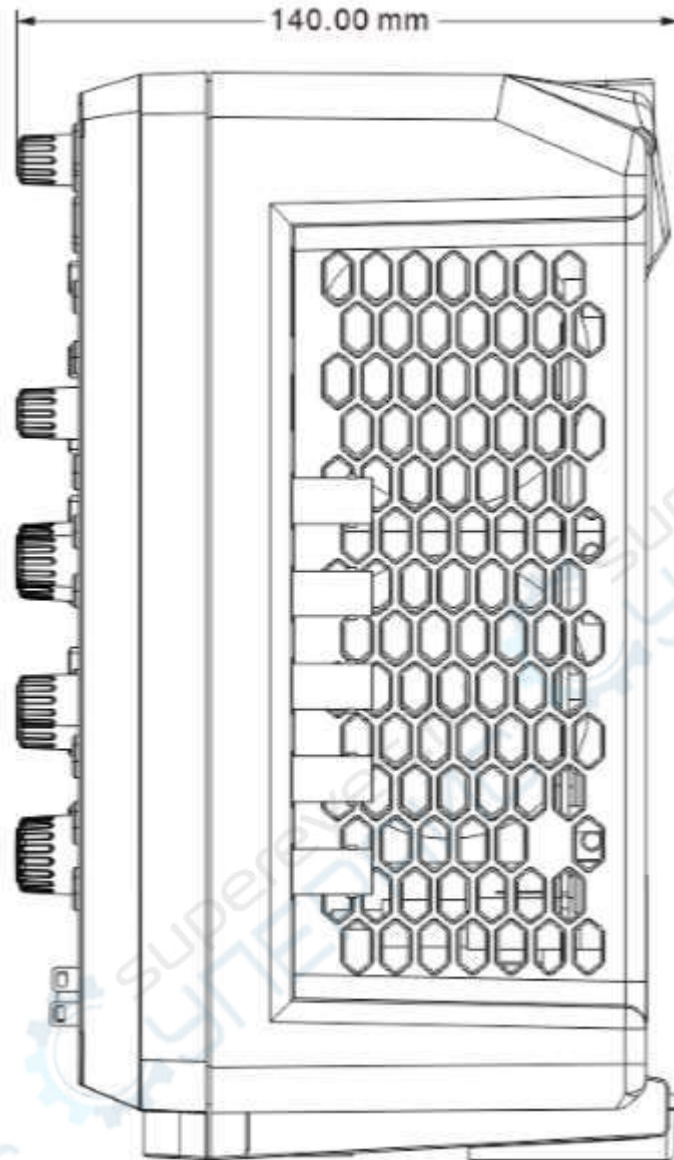
图 4.2 侧视图
