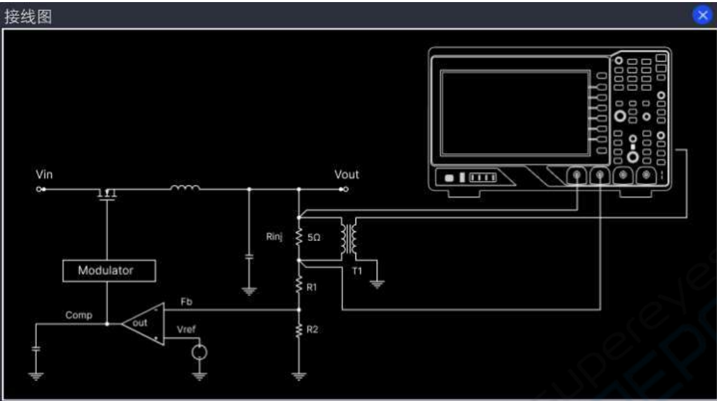
图 16.3 波特图接线图
