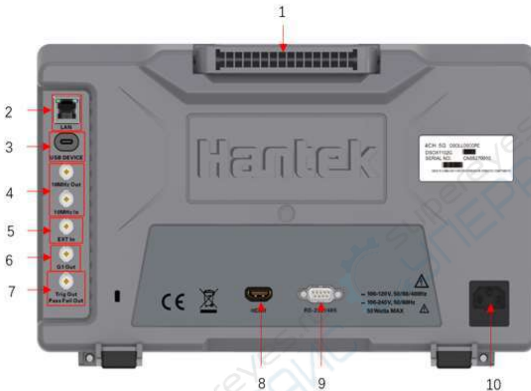
图 4.9 后面板总览图
