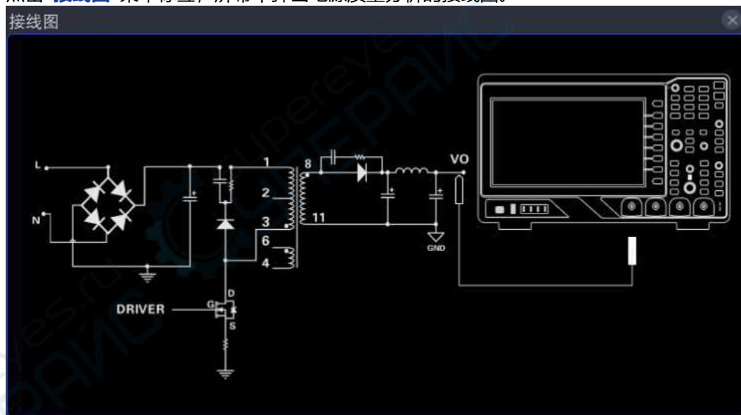
图 16.2 纹波接线图
