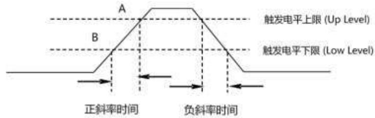
图 8.5 正斜率/负斜率
