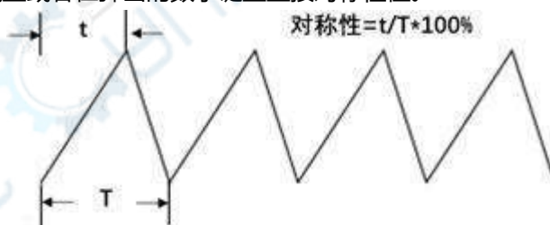
图 20.4 对称性定义
