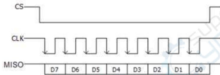
图 8.13 SPI 触发示意图
