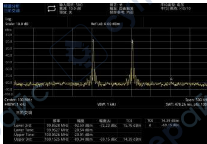
图 5-4：三阶交调
