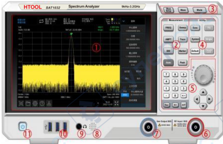
图 1-1：前面板
