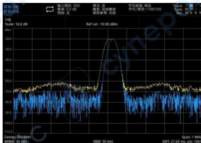
图 3-15：用最大保持和刷新来观察信号飘移
