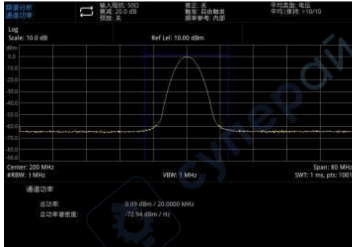
图 5-1：通道功率
