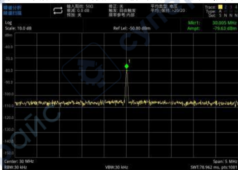
图 3-14：迹线平均
