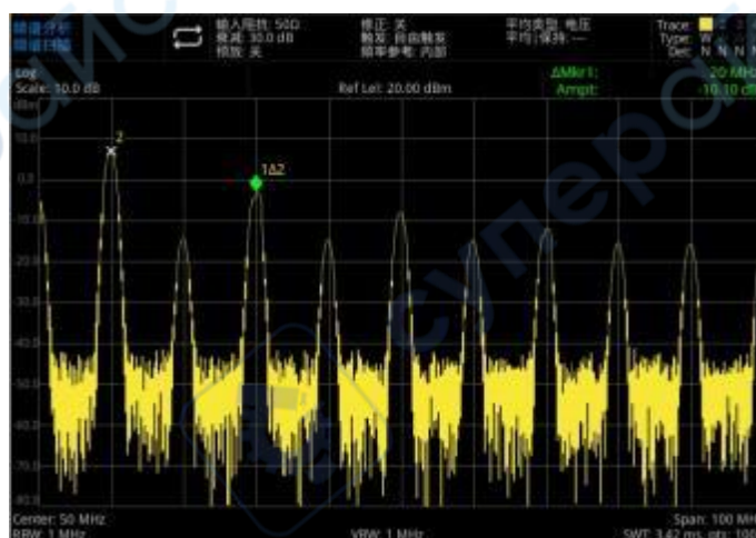
图 3-2：标记模式差值 △ 在同一屏幕信号比较
