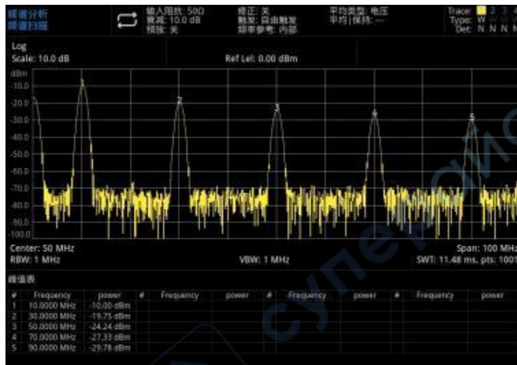
图 4-3：峰值表
