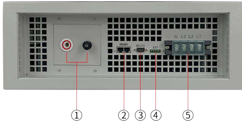
①输出接口 ②RS-485 通信接口 ③RS-232 通信接口 ④外部采样控制接口 ⑤市电输入口
