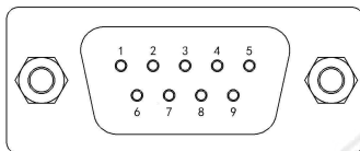
接口示意图
