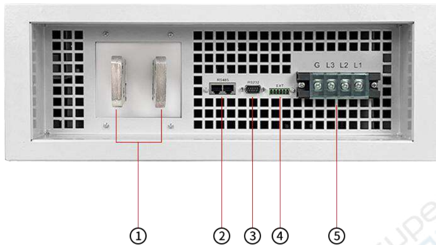
图 7 机架式电源接口面板
