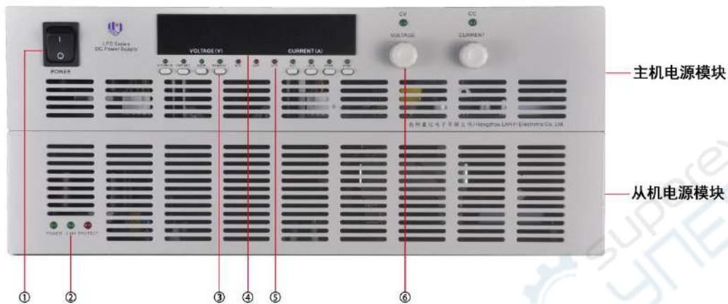
图 5 电源前面板（以 10KW 为例）
