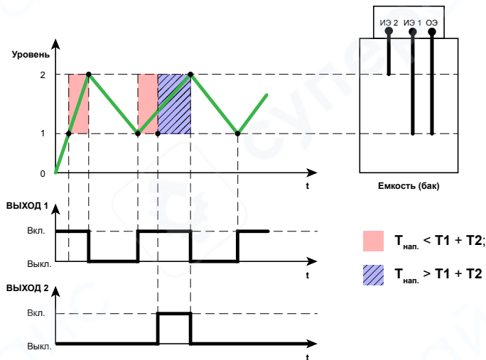
Рисунок 6.8 – График работы алгоритма А-2.2 «Наполнение»
