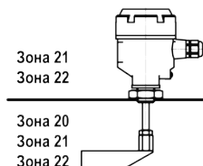
Рисунок 1.1 – Классы взрывоопасных зон работы PCY
