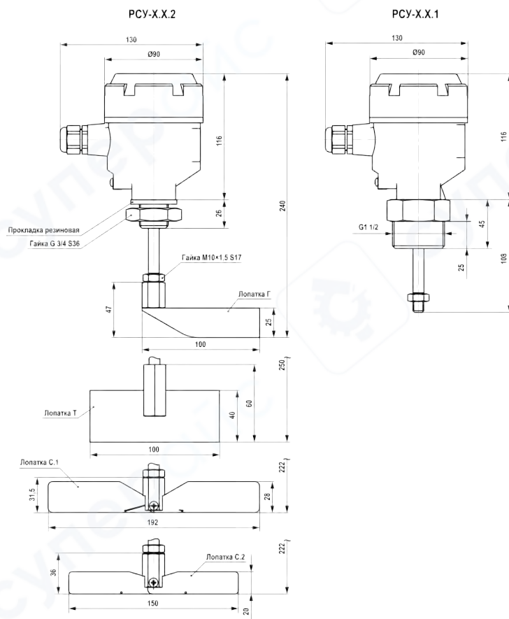
Рисунок 4.1 – Габаритные размеры PCY
