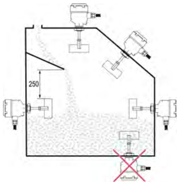
Рисунок 4.2 – Расположение на объекте
