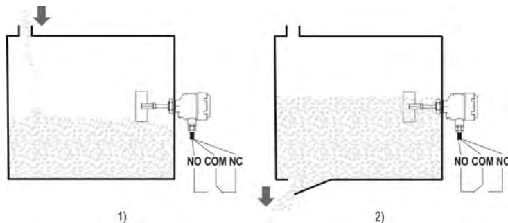
Рисунок 6.1 – Срабатывание микропереключателя: на наполнение (1); на опустошение (2)
