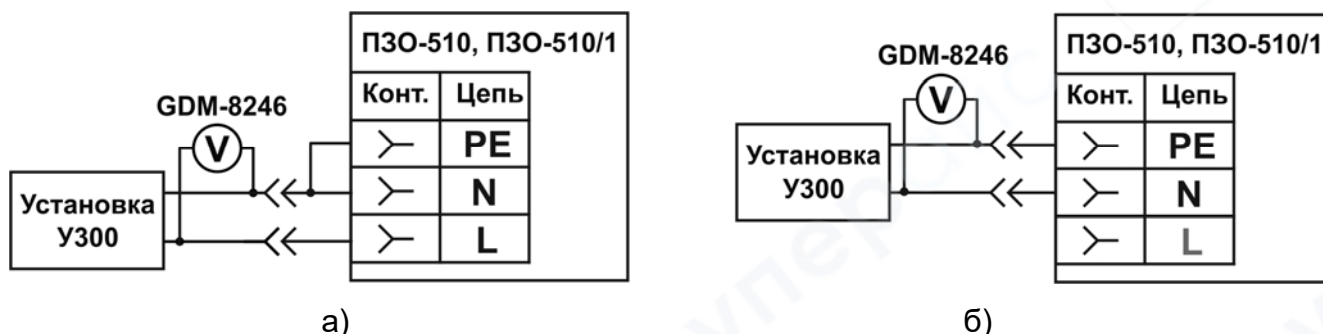
Рисунок 6.7.1 – Схемы проверки погрешности измерений напряжения переменного тока
