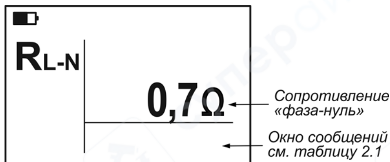
Рисунок 2.10 – Показания при измерении сопротивления петли «фаза-нуль»
