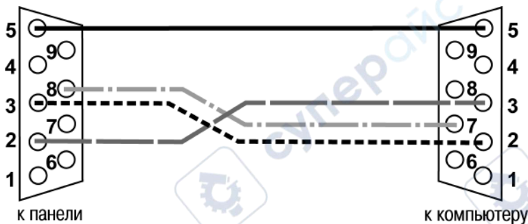
Рисунок В.1 - Соединительный нуль-модемный кабель для конфигурирования панели ИР320 с переходником
