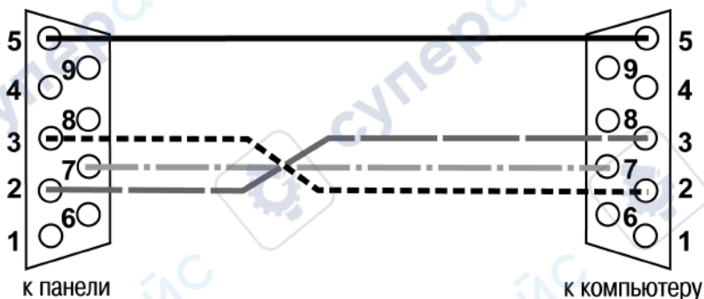
Рисунок В.2 - Соединительный кабель для конфигурирования панели ИР320 без переходника
