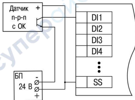
Рисунок 5.7 – Подключение транзисторов п-р-п
