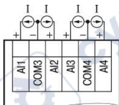
Рисунок 6.4 – Схема подключения активного датчика с выходом типа «Ток 4...20 мА»
