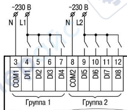
Рисунок 6.2 – Схема подключения дискретных датчиков с питанием 230 В
