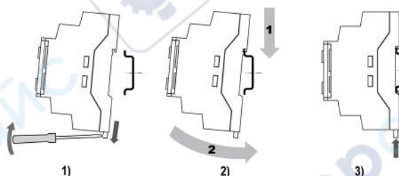
Рисунок 5.1 – Монтаж и демонтаж прибора
