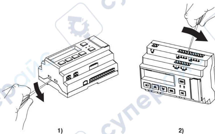
Рисунок 8.1 – Снятие верхней крышки
