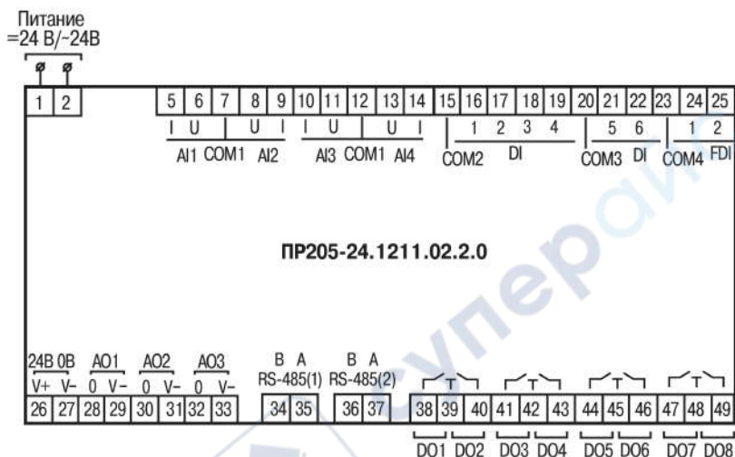
Рисунок А.6 – Расположение контактов для ПР205-24.1211.02.2.0
