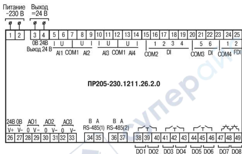
Рисунок А.2 – Расположение контактов для ПР205-230.1211.22.2.0
