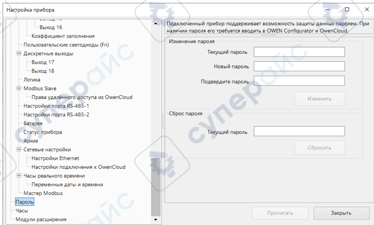
Рисунок 4.19 – Пароль доступа
