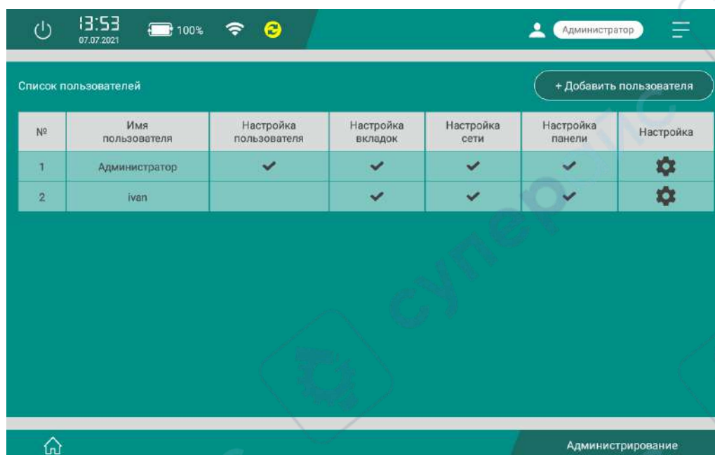
Рисунок 7.4 – Вкладка «Администрирование»
