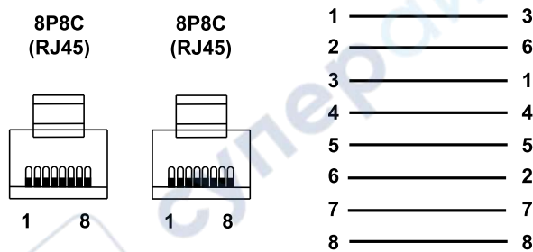
Рисунок 5.4 – Схема перекрестного кабеля для соединения прибора по сети Ethernet
