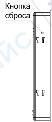
Рисунок 7.1 – Кнопка сброса
