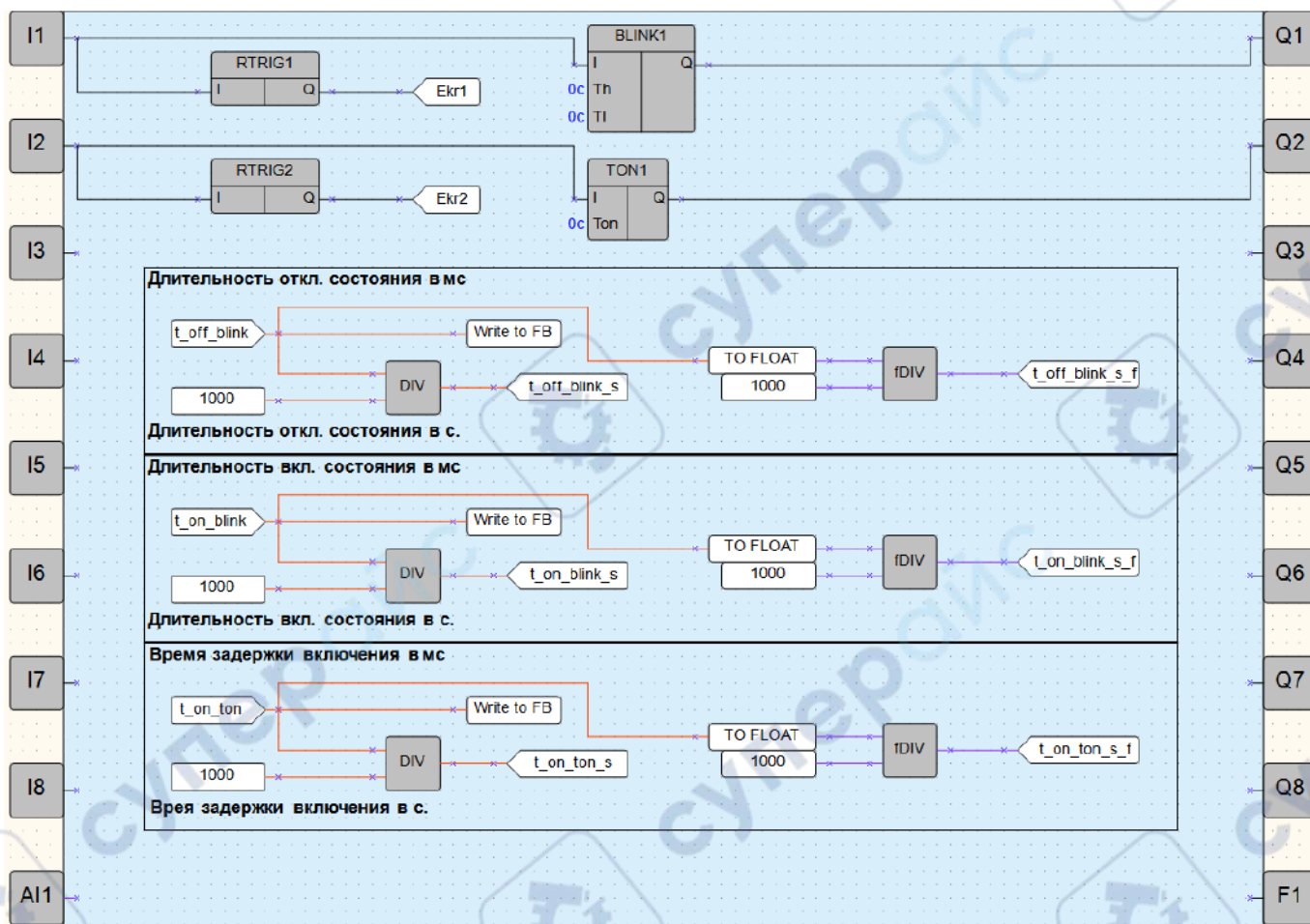
Рисунок 11.12 – Схема алгоритма
