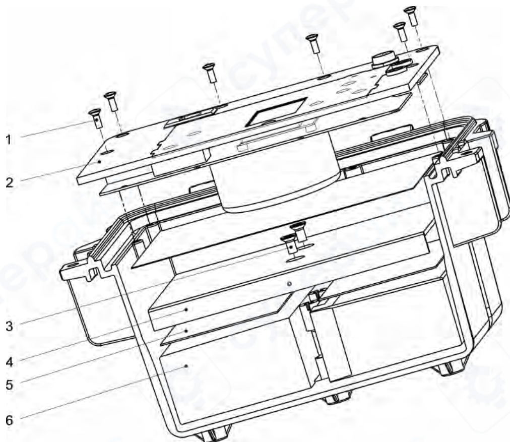
Рисунок 3.1 – Замена аккумуляторов
