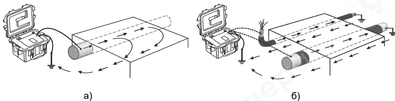
Рисунок 2.3 –Подключение генератора к коммуникациям:
