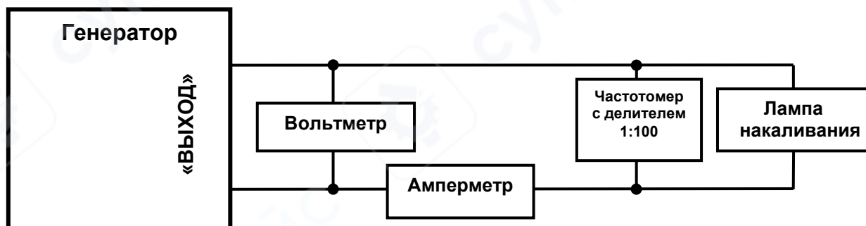
Рисунок 7.5.2 – Схема рабочего места для проверки параметров генератора
