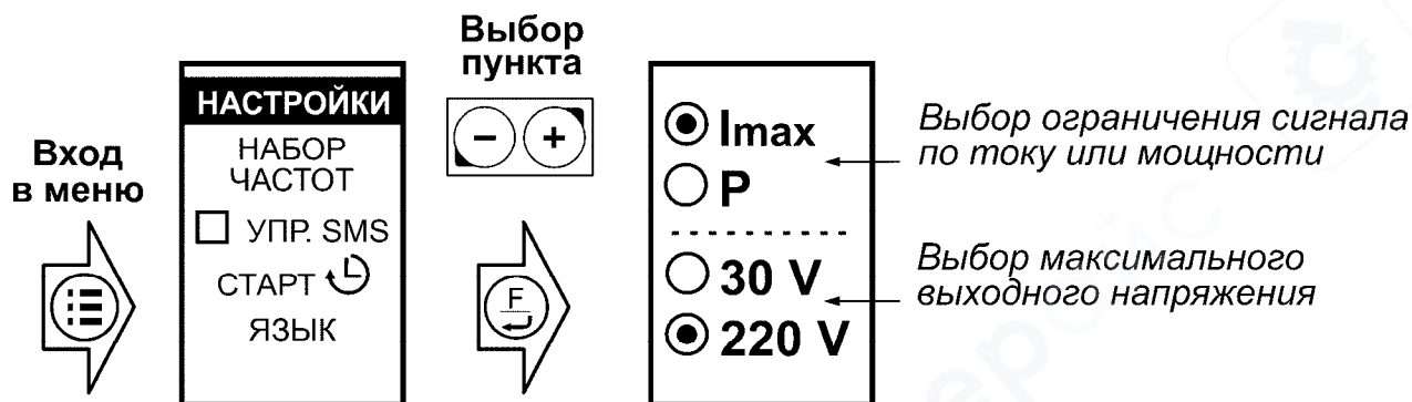
Рисунок 2.1 – Меню. Настройки генератора
