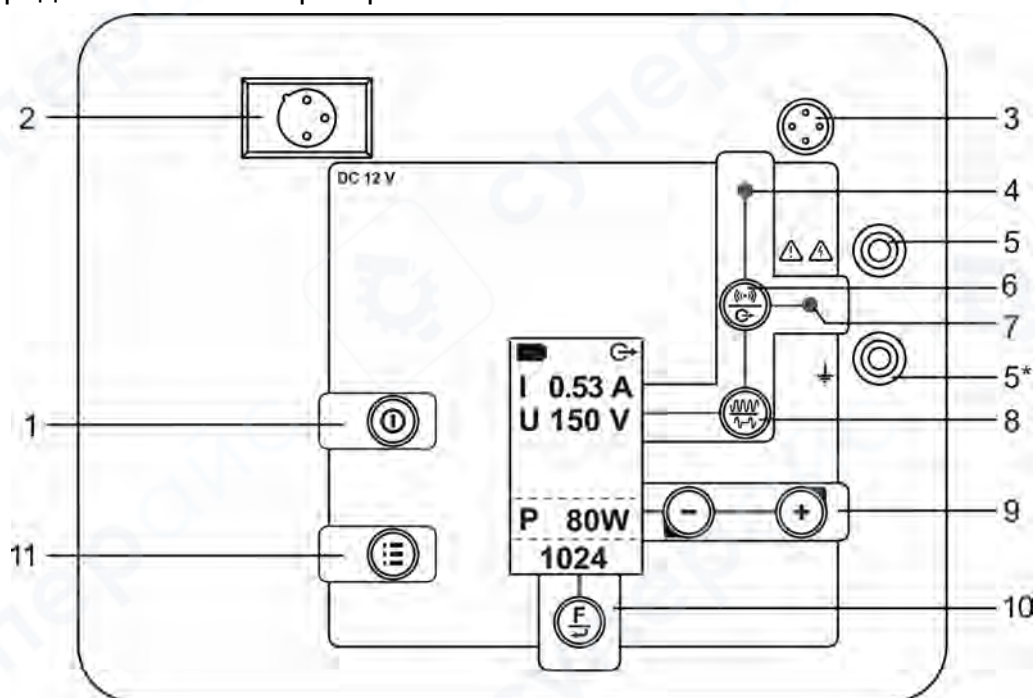
Рисунок 1.2 - Передняя панель генератора
