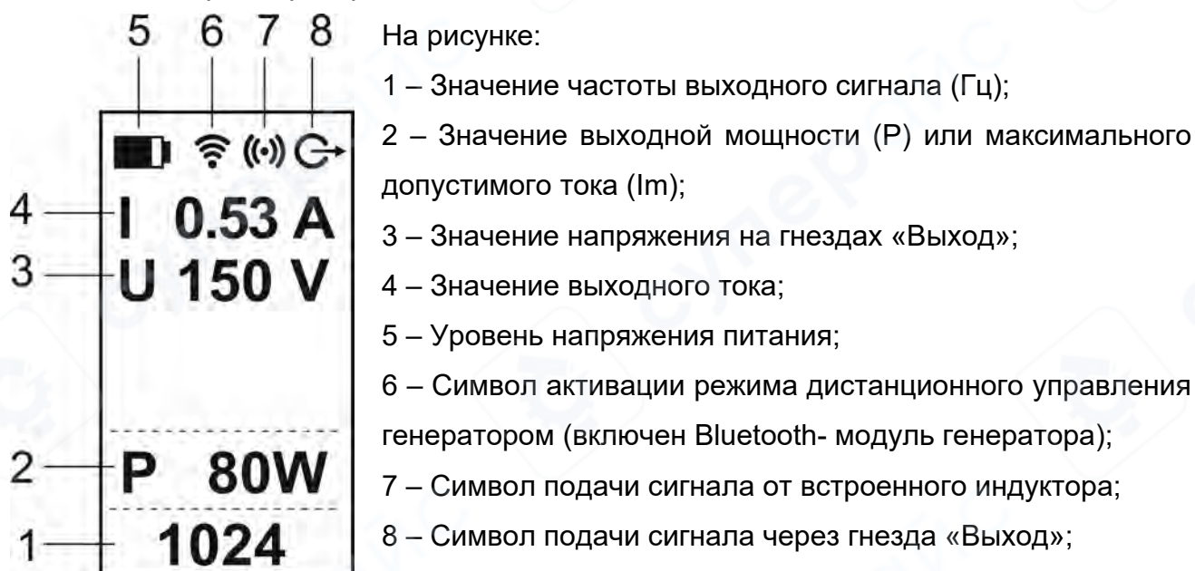
Рисунок 1.3 - Индикатор генератора
