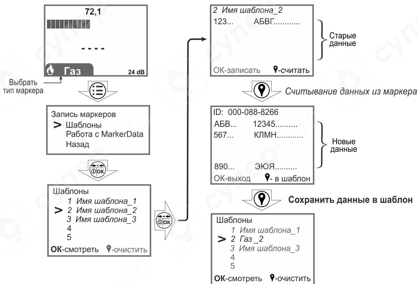
Рисунок 4.2.4 – Считывание данных из маркера в шаблон
