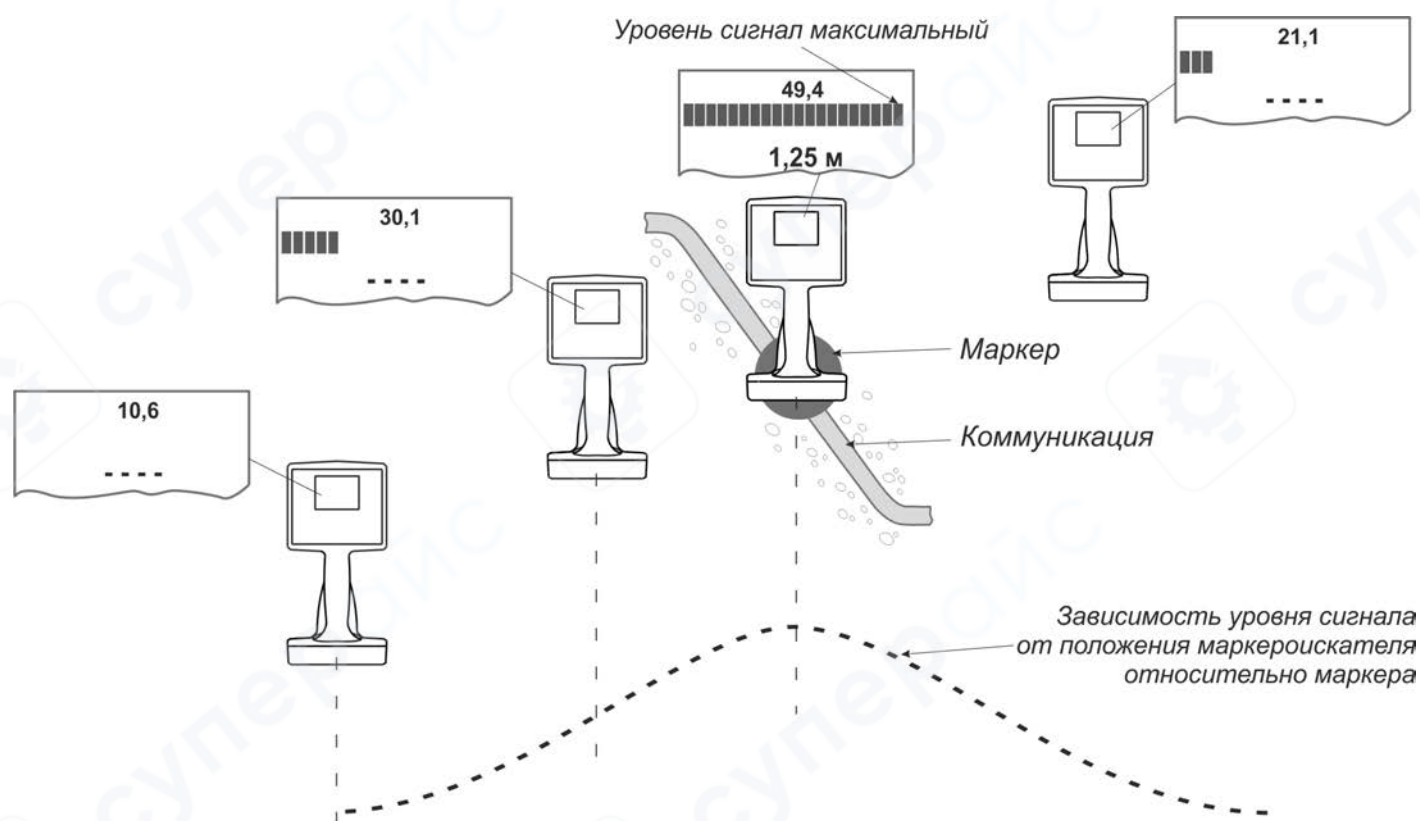
Рисунок 3.2 б – Зависимость уровня сигнала от положения маркероискателя
