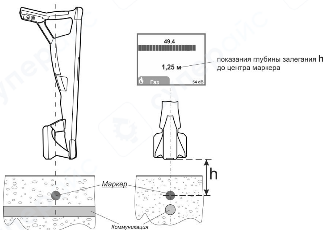
Рисунок 3.2 в – Определение глубины залегания
