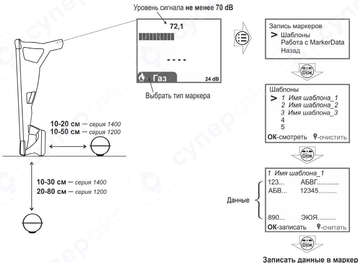
Рисунок 4.2.3а – Запись маркеров
