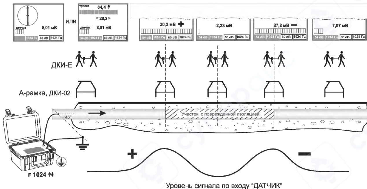
Рисунок 5.2.1 – Схема подключения и уровень сигнала при поиске повреждения изоляции по падению сигнала со сменой знака
